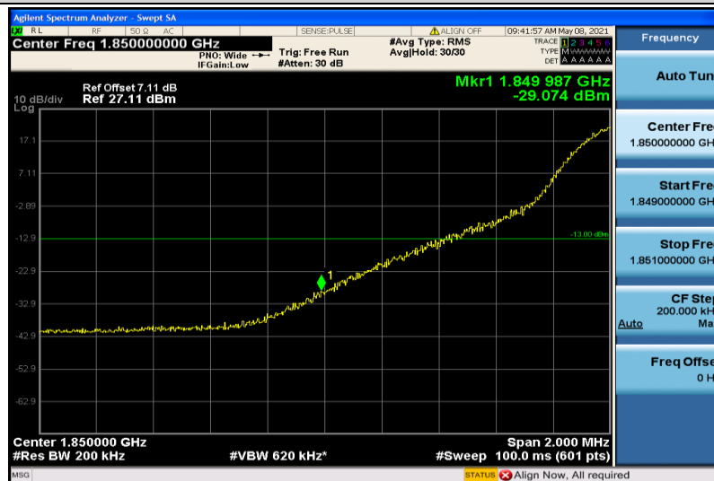
Band25-20MHz-QPSK-26140-1RB#0
