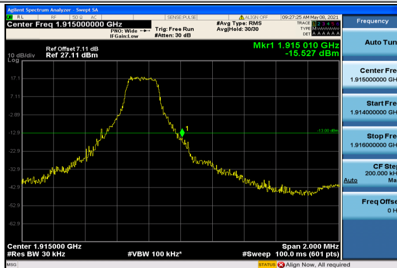
Band25-3MHz-QPSK-26675-1RB#14
