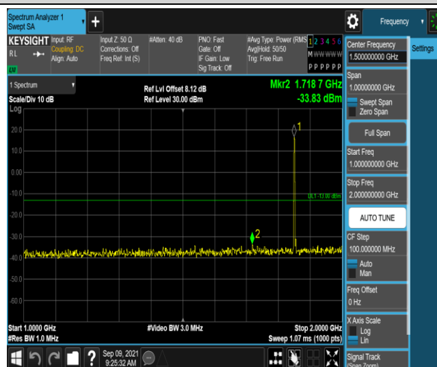
Band2-3MHz-QPSK-18615-1RB#0-Range4:1000~2000MHz
