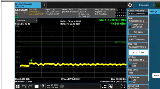
Band26(824-849)-10MHz-QPSK-26990-1RB#0-3000~10000-PAS
