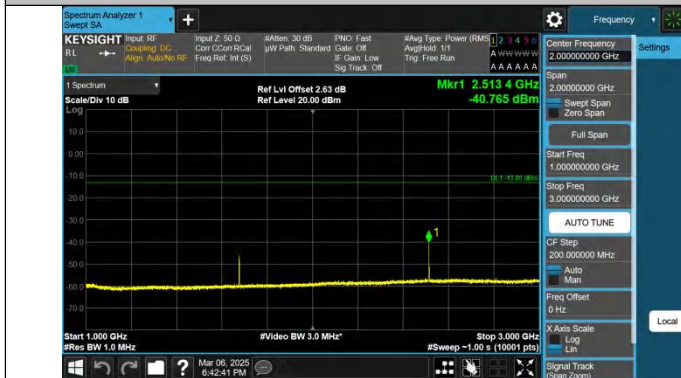
Band26(824-849)-3MHz-QPSK-26915-1RB#14-1000~3000-PASS
