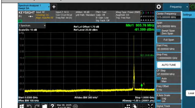
Band26(824-849)-3MHz-QPSK-27025-1RB#0-30~1000-PASS
