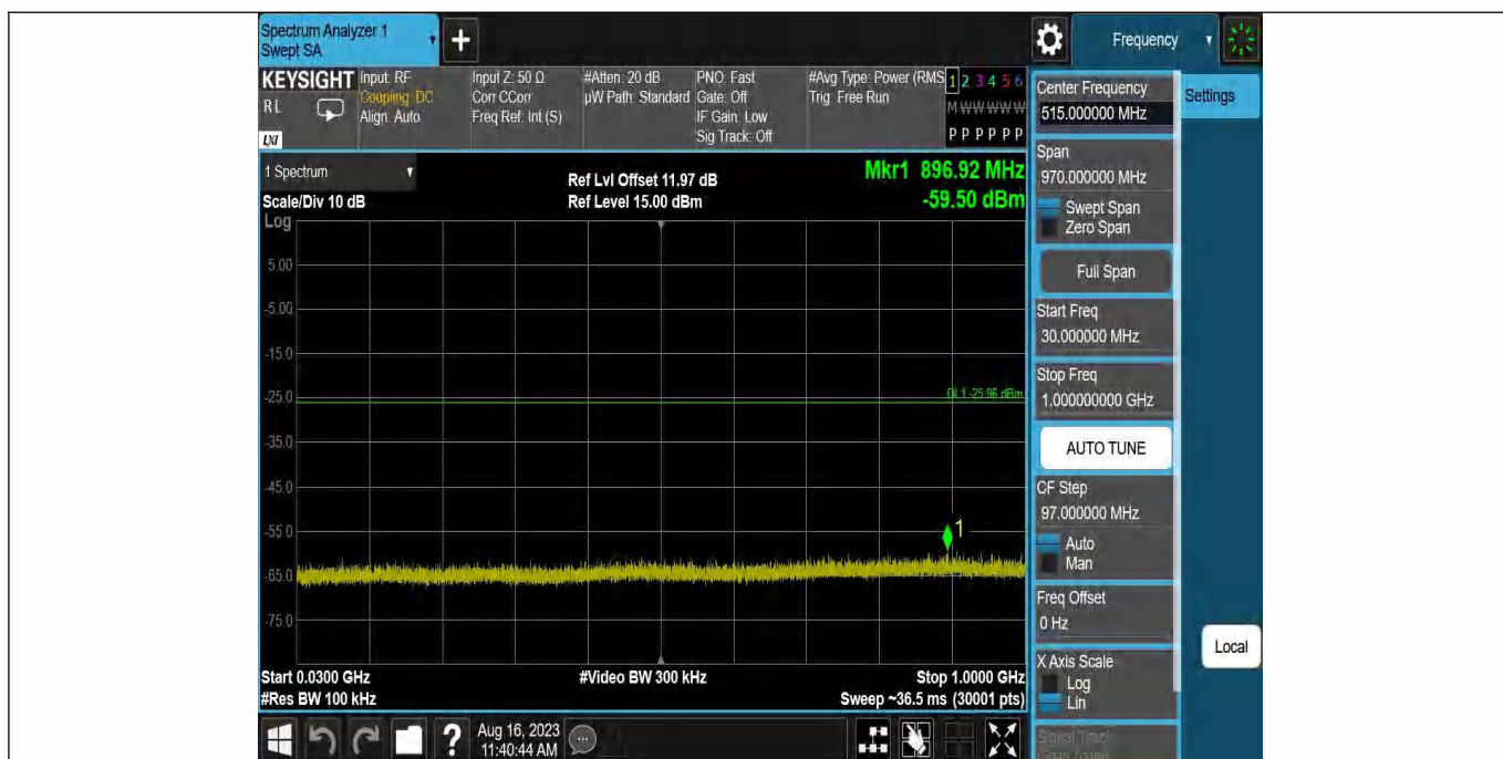
DH5-Ant1-2441-30~1000
