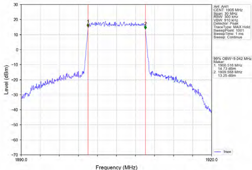
Band2_10MHz_QPSK_HCH_1905MHz_RB_50_0_NTNV
