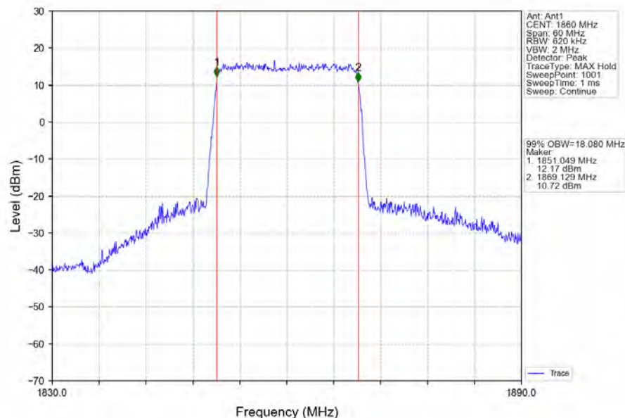
Band2_20MHz_64QAM_LCH_1860MHz_RB_100_0_NTNV
