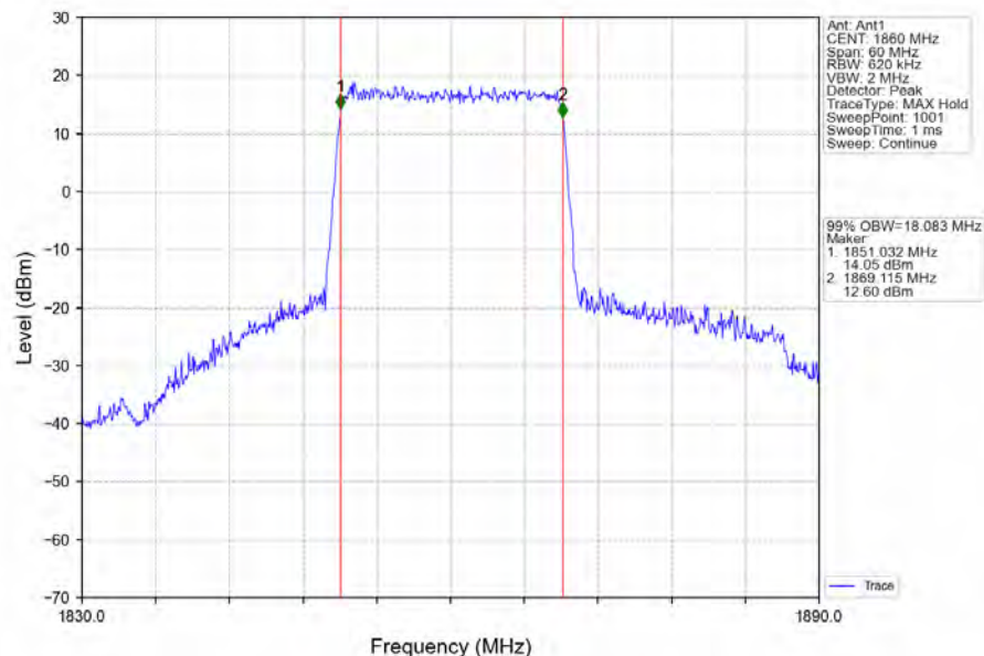
Band2_20MHz_QPSK_LCH_1860MHz_RB_100_0_NTNV
