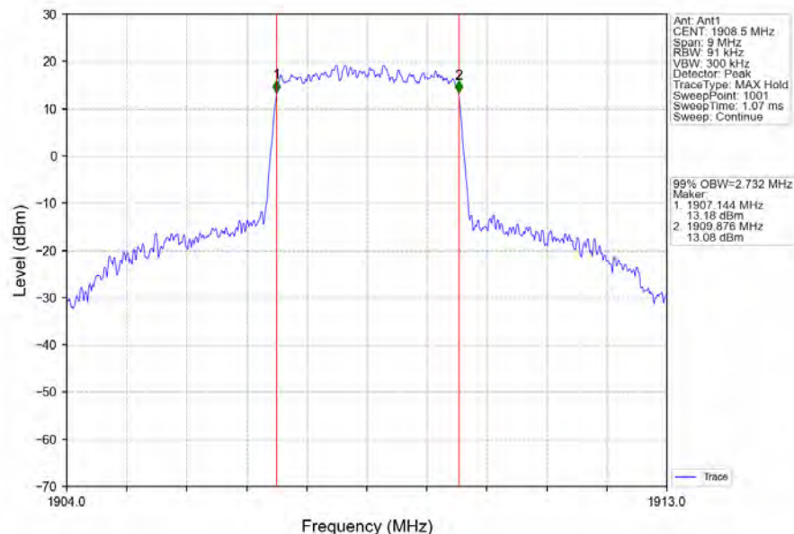
Band2_3MHz_QPSK_HCH_1908.5MHz_RB_15_0_NTNV
