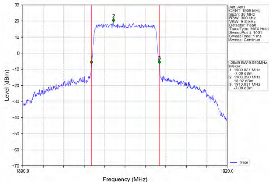
Band2_10MHz_QPSK_HCH_1905MHz_RB_50_0_NTNV
