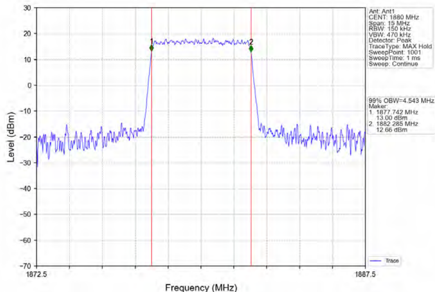
Band2_5MHz_QPSK_MCH_1880MHz_RB_25_0_NTNV
