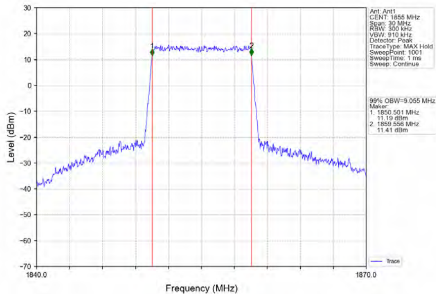
Band2_10MHz_64QAM_LCH_1855MHz_RB_50_0_NTNV
