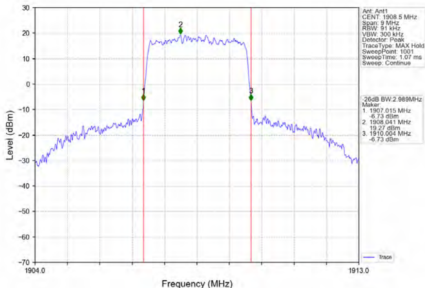
Band2_3MHz_QPSK_HCH_1908.5MHz_RB_15_0_NTNV
