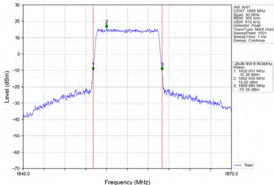
Band2_10MHz_64QAM_LCH_1855MHz_RB_50_0_NTNV
