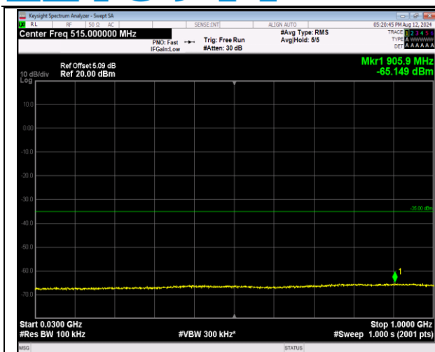
7-7-20MHz-10MHz-QPSK-QPSK-20850-20994-100RB# 0-50RB#0-30~1000MHz-PASS
