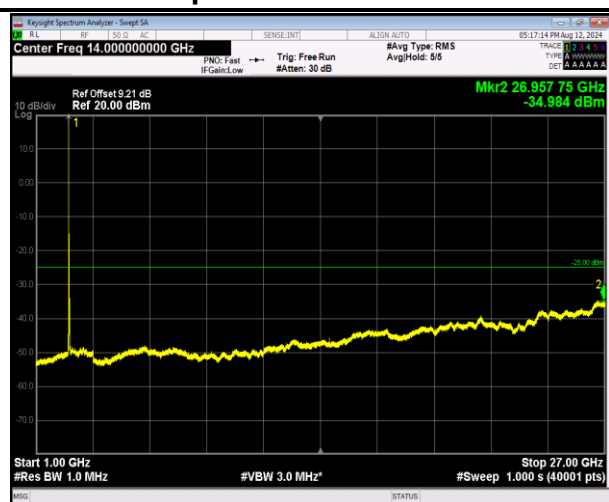
7-7-20MHz-10MHz-QPSK-QPSK-20850-20994-1RB#0-0 RB#0-1000~27000MHz-PASS
