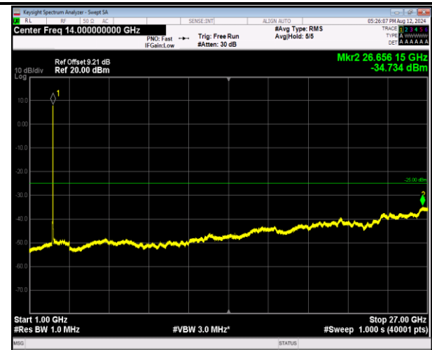
7-7-20MHz-10MHz-QPSK-QPSK-21051-21195-100RB#0-50RB#0-1000~27000MHz-PASS
