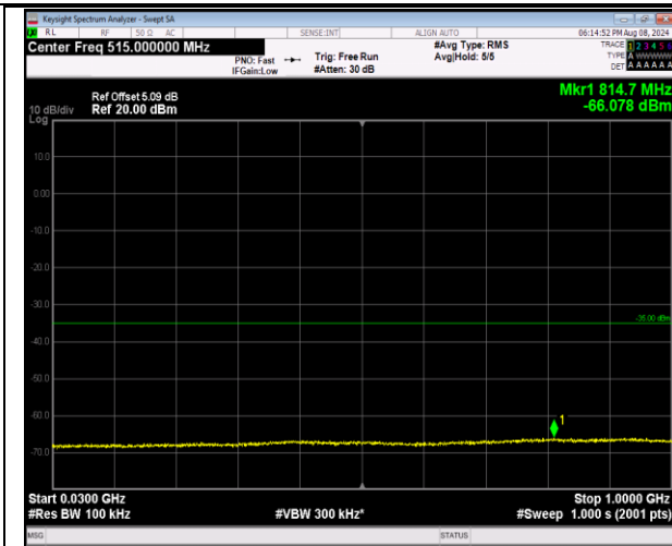
7-7-10MHz-20MHz-QPSK-QPSK-20805-20949-50RB#0-100RB#0-30~1000MHz-PASS
