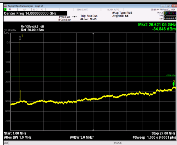
7-7-20MHz-10MHz-QPSK-QPSK-20850-20994-1RB#0-1 RB#49-1000~27000MHz-PASS
