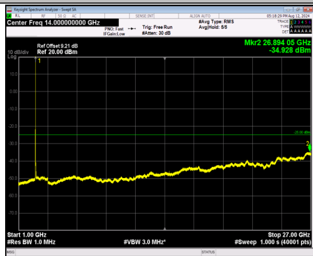
7-7-20MHz-10MHz-QPSK-QPSK-20850-20994-1RB#99-0 RB#0-1000~27000MHz-PASS
