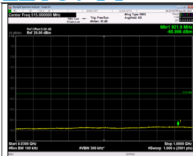
7-7-10MHz-20MHz-QPSK-QPSK-21206-21350-50RB#0-100RB#0-30~1000MHz-PASS
