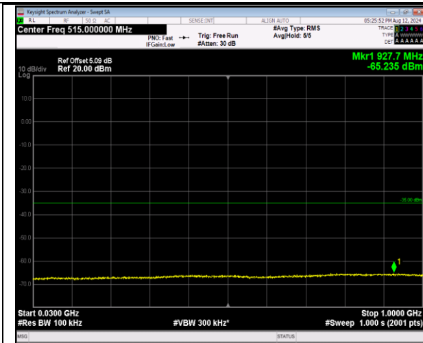
7-7-20MHz-10MHz-QPSK-QPSK-21051-21195-100RB#0-50RB#0-30~1000MHz-PASS
