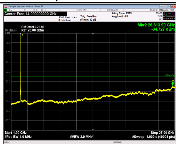
7-7-20MHz-10MHz-QPSK-QPSK-21051-21195-1RB#0-0 RB#0-1000~27000MHz-PASS
