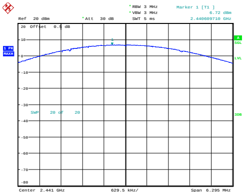
\pi/4 -DQPSK_Middle 6.72dBm
