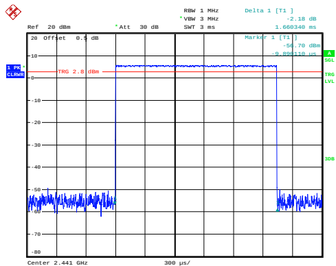
GFSK_Hopping_DH3 1.660ms
