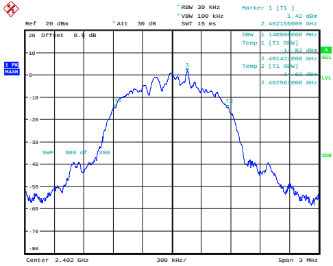
\pi/4 -DQPSK_Low 1.140MHz
