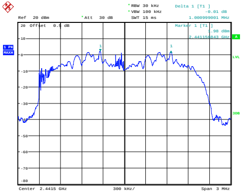
\pi/4 -DQPSK_Middle 1.001MHz
