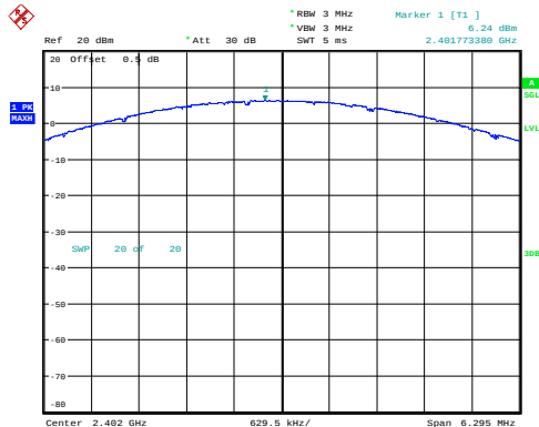
\pi/4 -DQPSK_Low 6.24dBm
