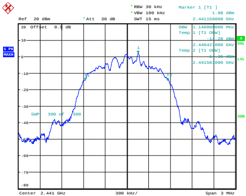
\pi/4 -DQPSK_Middle 1.140MHz
