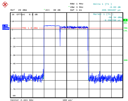
\pi/4 -DQPSK_Hopping_2DH1 0.407ms
