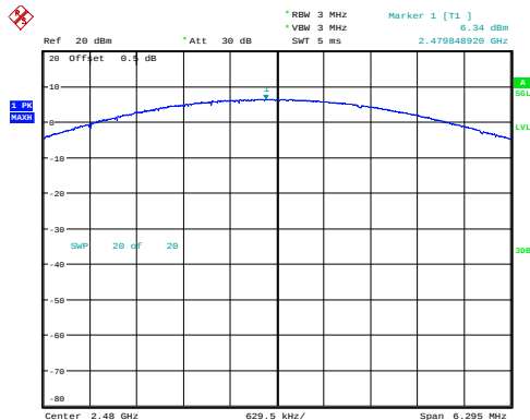
\pi/4 -DQPSK_High 6.34dBm
