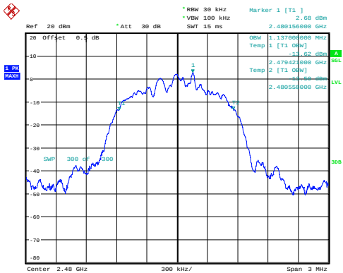
\pi/4 -DQPSK_High 1.137MHz
