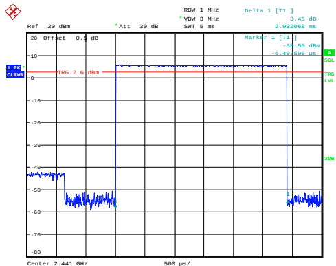
GFSK_Hopping_DH5 2.932ms
