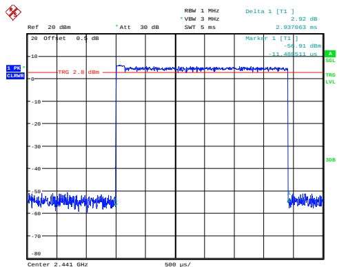
\pi/4 -DQPSK_Hopping_2DH5 2.937ms
