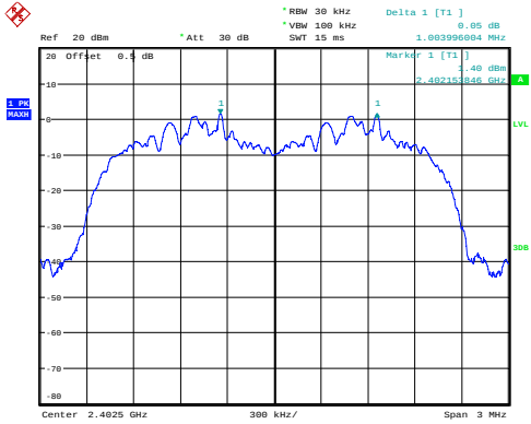
\pi/4 -DQPSK_Low 1.004MHz
