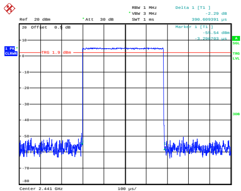
GFSK_Hopping_DH1 0.391ms
