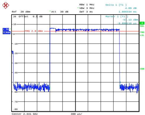
\pi/4 -DQPSK_Hopping_2DH3 1.666ms
