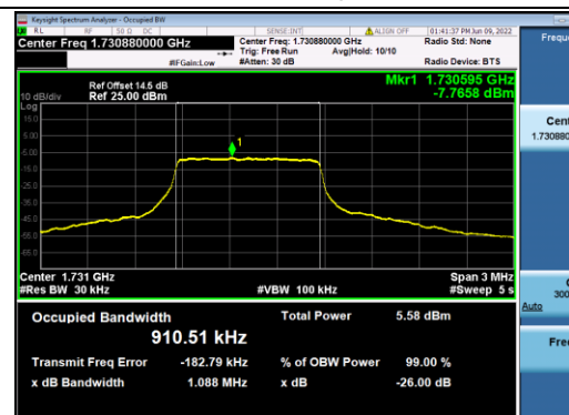
B4-5M-Mid CH-OBW-Q16
