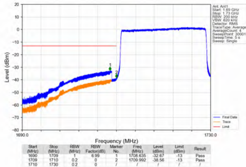
Band4_20MHz_256QAM_LCH_1720MHz_RB_100_0_NTNV
