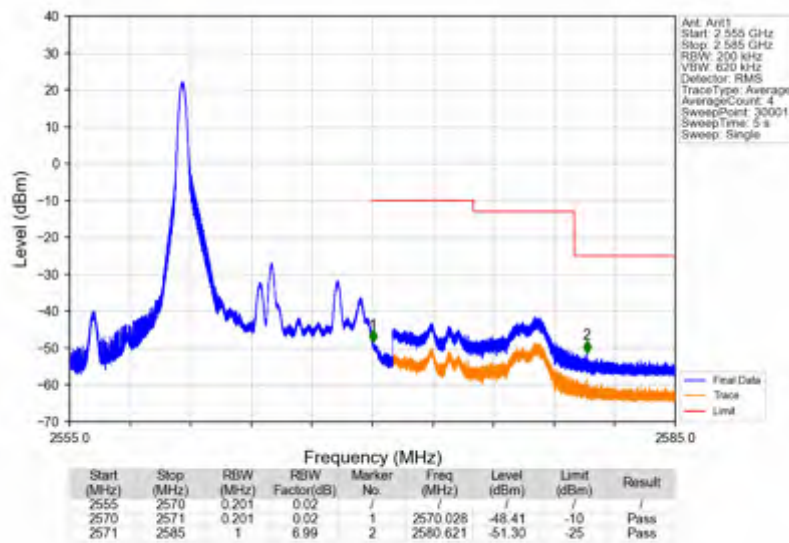
Band7_10MHz_QPSK_HCH_2565MHz_RB_50_0_NTNV
