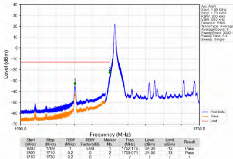
Band4_20MHz_QPSK_LCH_1720MHz_RB_1_0_NTNV
