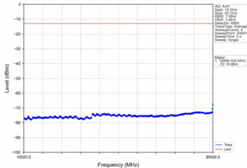
Band4_20MHz_256QAM_LCH_1720MHz_RB_100_0_NTNV
