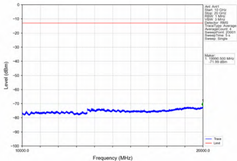
Band4_20MHz_QPSK_LCH_1720MHz_RB_100_0_NTNV
