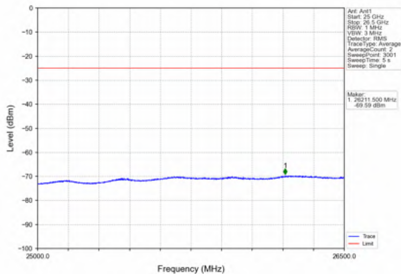
Band7_5MHz_QPSK_HCH_2567.5MHz_RB_1_24_NTNV
