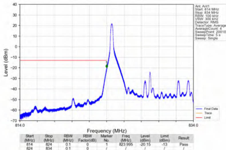
Band5_10MHz_QPSK_LCH_829MHz_RB_1_0_NTNV
