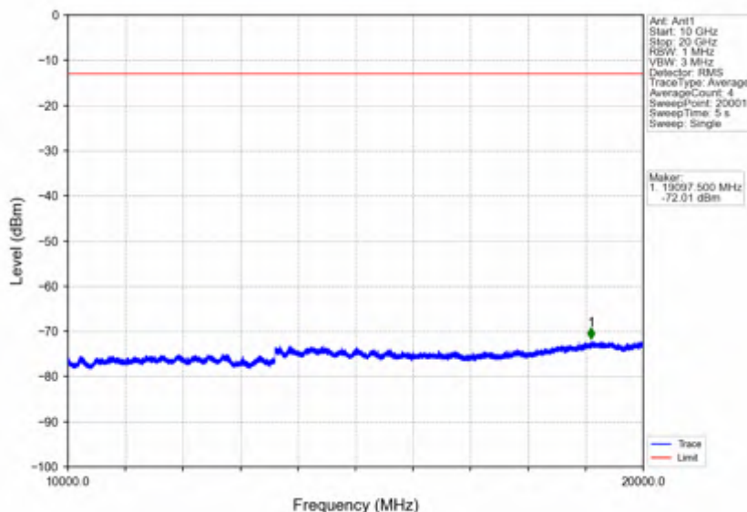
Band4_20MHz_QPSK_HCH_1745MHz_RB_1_0_NTNV
