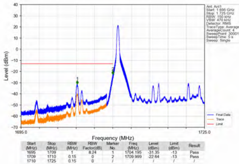
Band4_15MHz_QPSK_LCH_1717.5MHz_RB_1_0_NTNV
