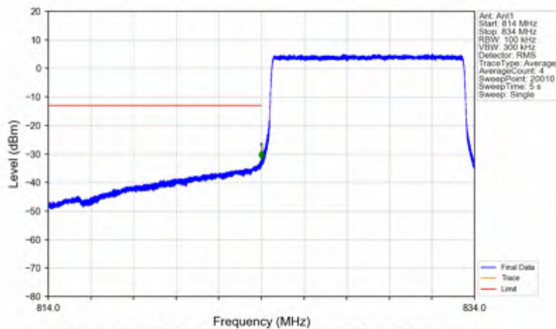
Band5_10MHz_QPSK_LCH_829MHz_RB_50_0_NTNV
