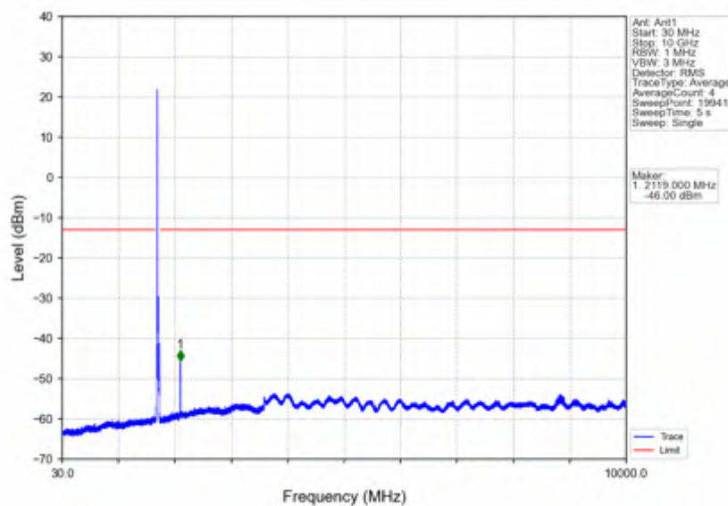
Band4_20MHz_16QAM_LCH_1720MHz_RB_1_0_NTNV
