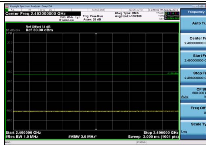
FDD07_20MHz_2560_QPSK_fullRB_ExtraBan ds_Range_2490~2496
