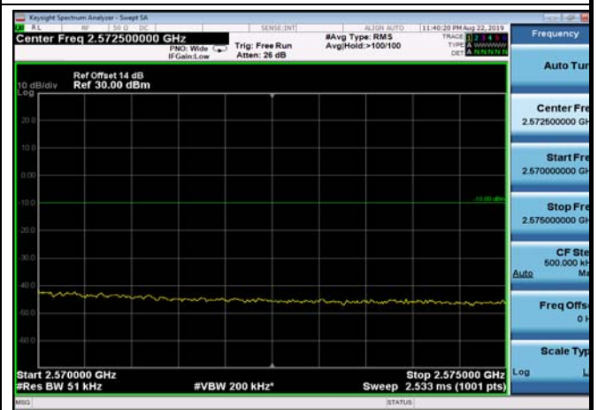
FDD07_20MHz_2560_QPSK_fullRB_ExtraBan ds_Range_2570~2575
