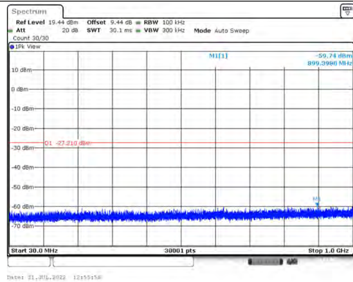
11B_Ant1_2412_30~1000
