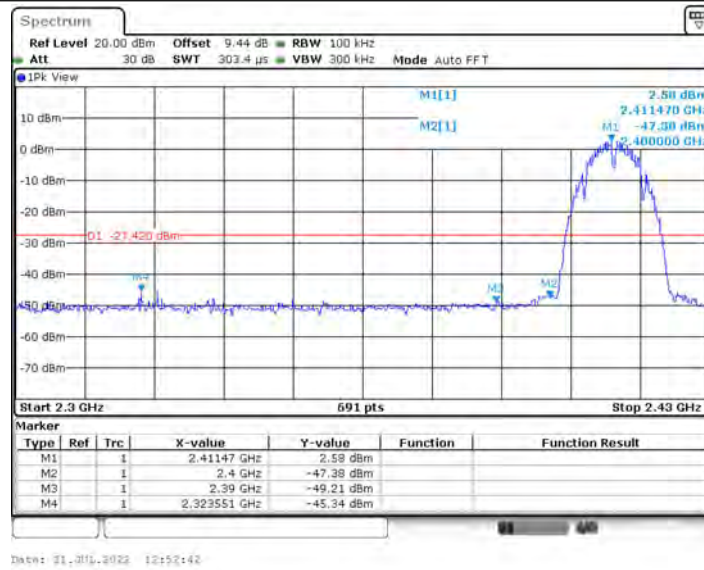
11B_Ant1_Low_2412
