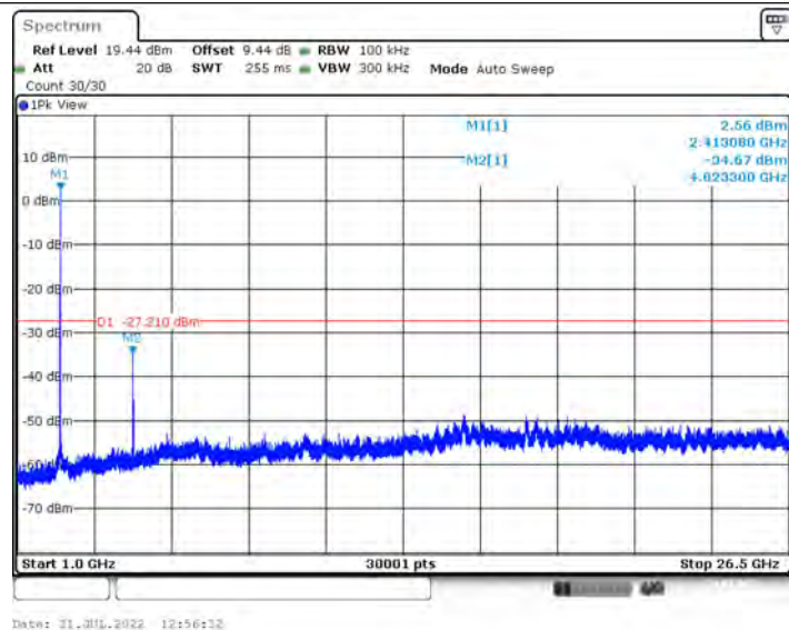
11B_Ant1_2412_1000~26500
