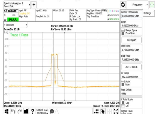
802.11be_80MHz_ChainA_6385MHz_484+242_MRUA3
