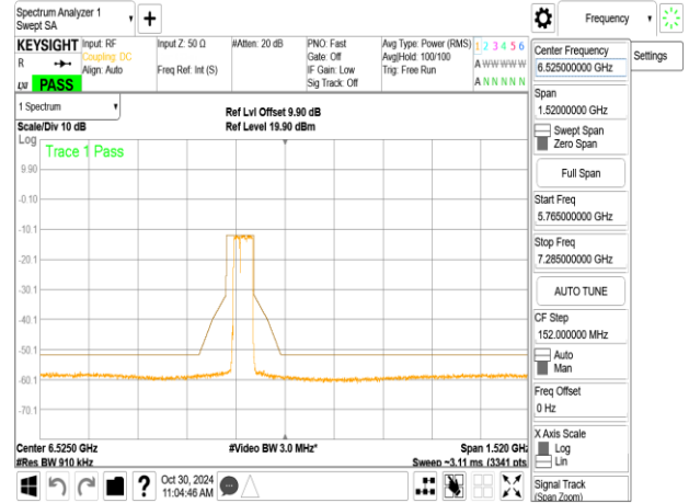
802.11be_80MHz_ChainA_6385MHz_484+242_MRUA3
