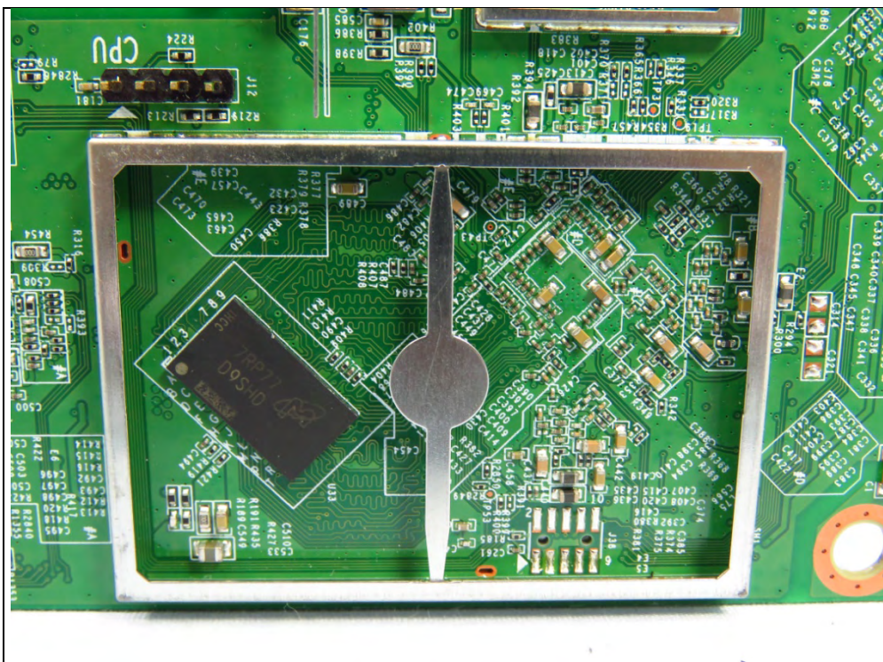
BT LE/ Zigbee Chip
