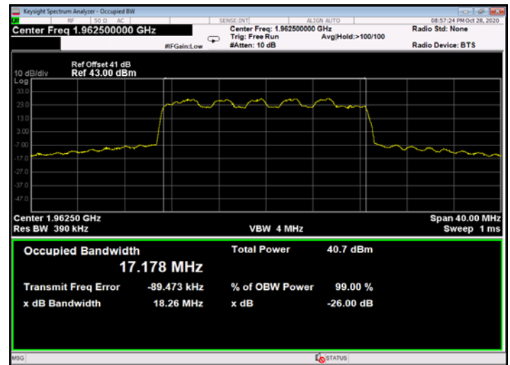
Figure 566: 16QAM 20MHz B.W.; 1962.5MHz, 60kHz - Output
