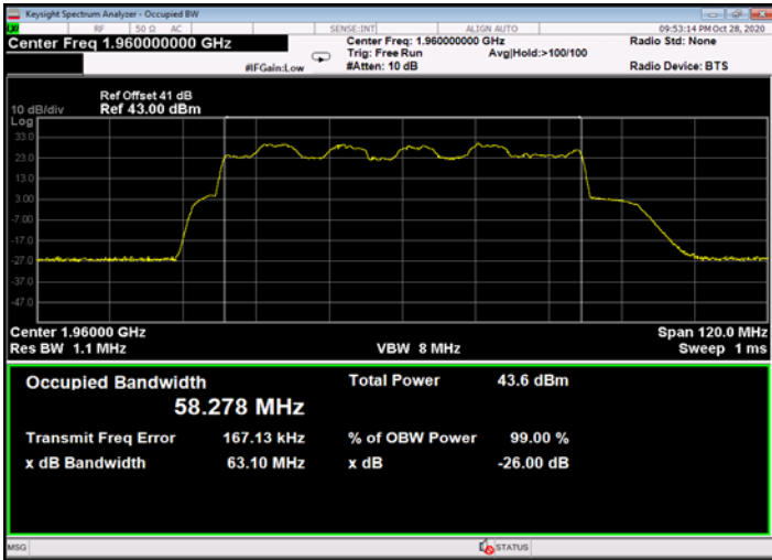
Figure 597: 16QAM 60MHz B.W.; 1960.0MHz, 30kHz - Output
