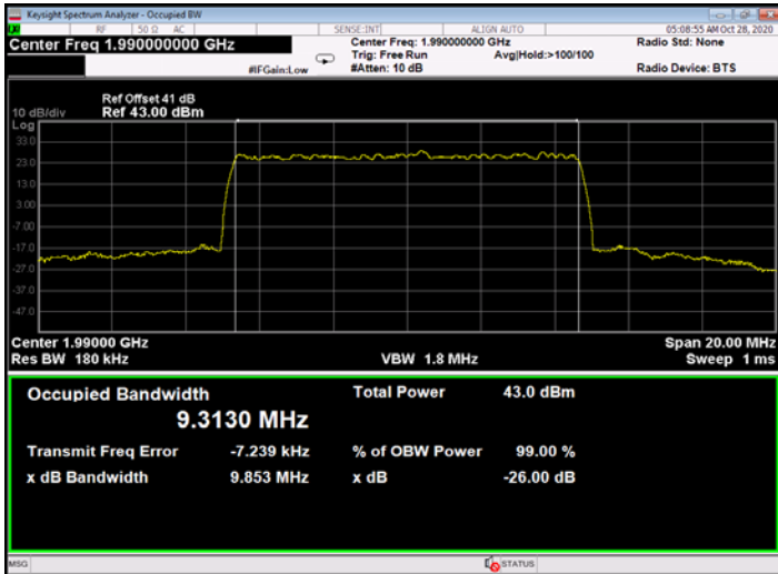
Figure 615: 64QAM 10MHz B.W.; 1990.0MHz, 15kHz - Output
