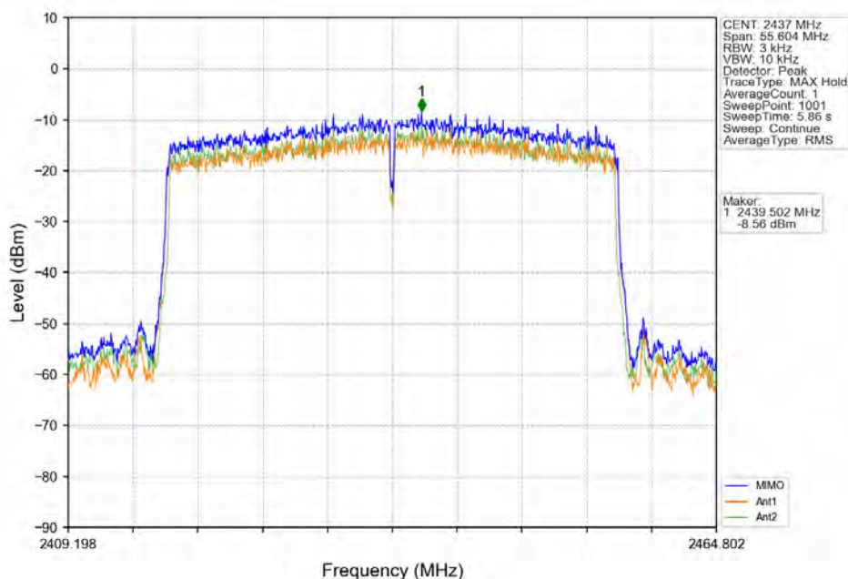
802.11ax(HE40) MCH_2437MHz_RU484_Left_MIMO_NTNV
