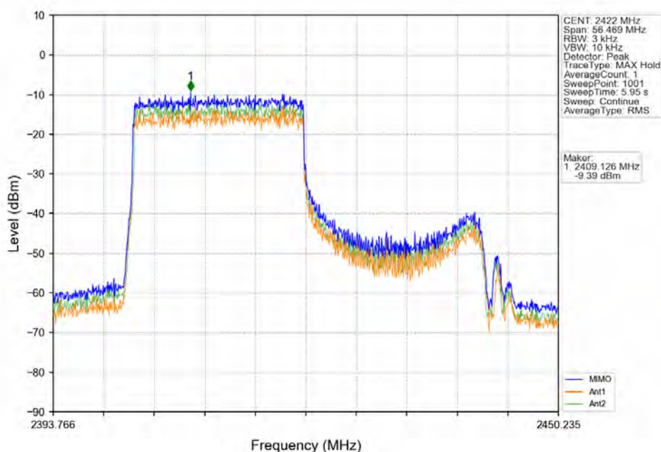
802.11ax(HE40) LCH_2422MHz_RU242_Left_MIMO_NTNV
