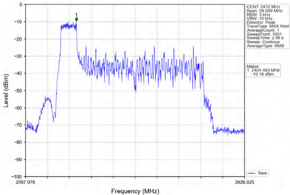
802.11ax(HE20)_LCH_2412MHz_RU26_Left_Ant1 (MIMO)_NTNV
