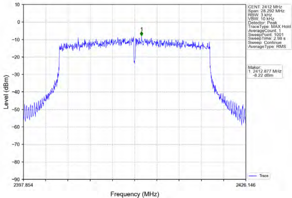
802.11ax(HE20) LCH_2412MHz_RU242_Left_Ant2 (MIMO) NTN
