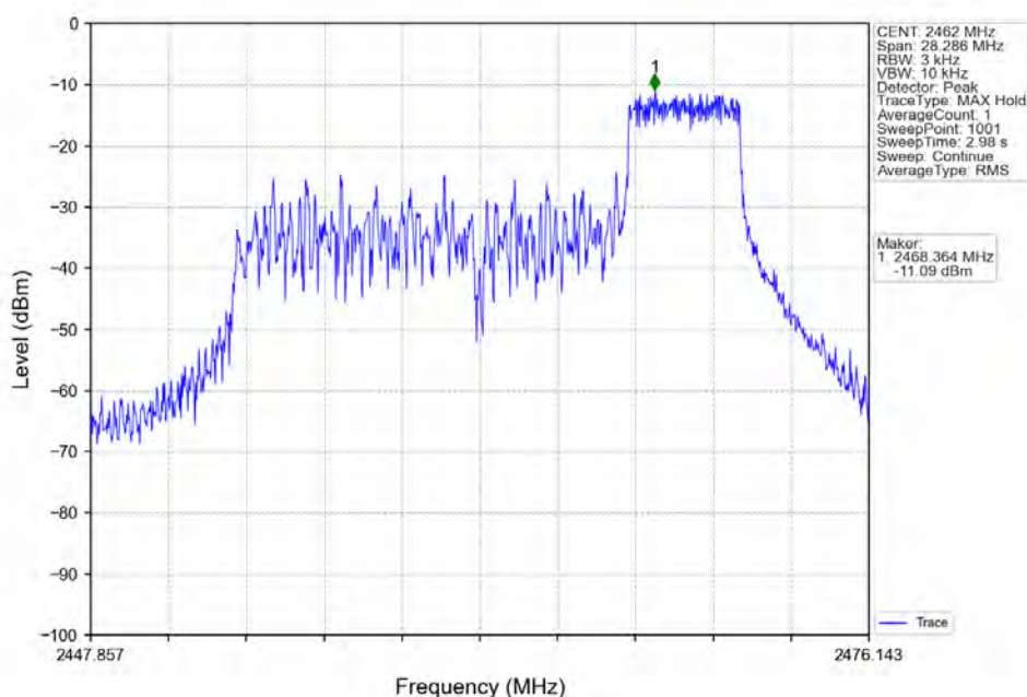
802.11ax(HE20)_HCH_2462MHz_RU52_Right_Ant1(MIMO)_NTNV
