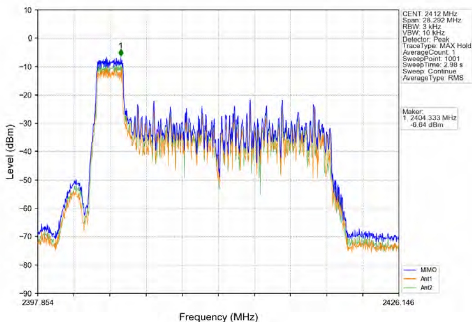
802.11ax(HE20)_LCH_2412MHz_RU26_Left MIMO_NTNV
