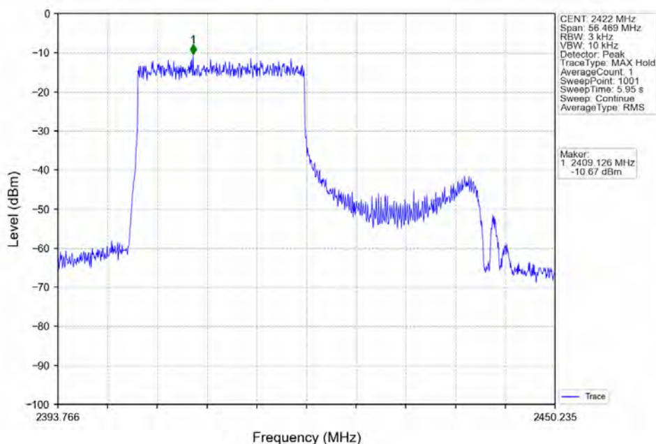
802.11ax(HE40) LCH_2422MHz_RU242_Left_Ant2 (MIMO) NTN
