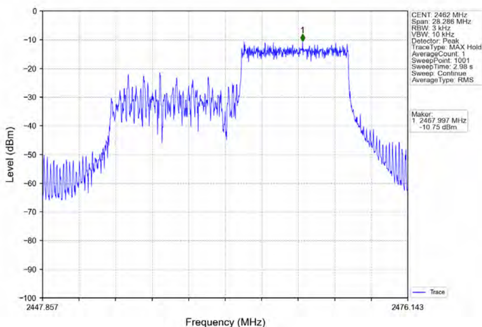
802.11ax(HE20)_HCH_2462MHz_RU106_Right_Ant1 (MIMO)_NTNV
