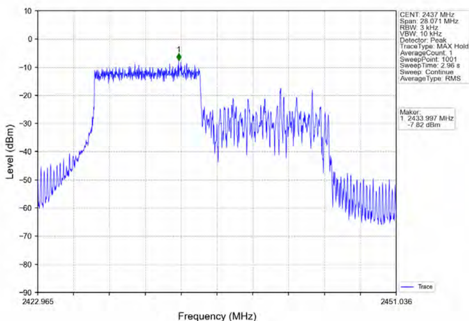
802.11ax(HE20)_MCH_2437MHz_RU106_Left_Ant2 (MIMO)_NTNV
