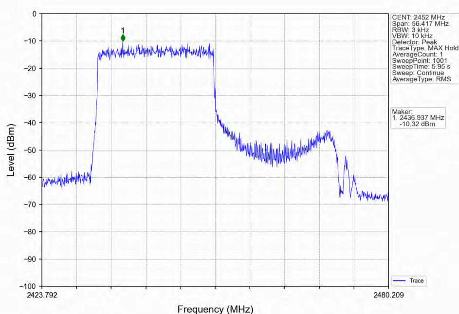
802.11ax(HE40)_HCH_2452MHz_RU242_Right_Ant2 (MIMO)_NTNV
