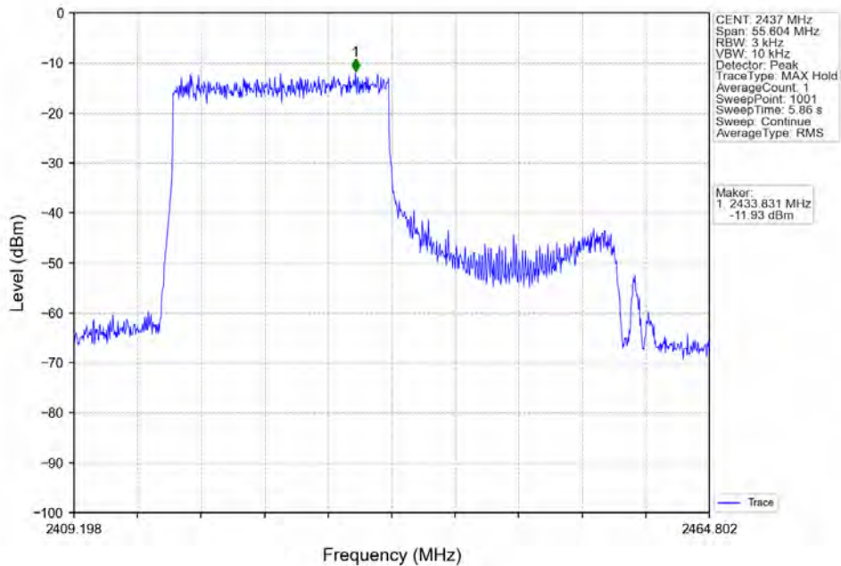
802.11ax(HE40)_MCH_2437MHz_RU242_Left_Ant2 (MIMO)_NTNV
