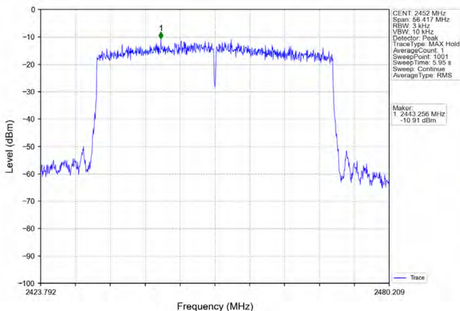
802.11ax(HE40)_HCH_2452MHz_RU484_Left_Ant2 (MIMO)_NTNV
