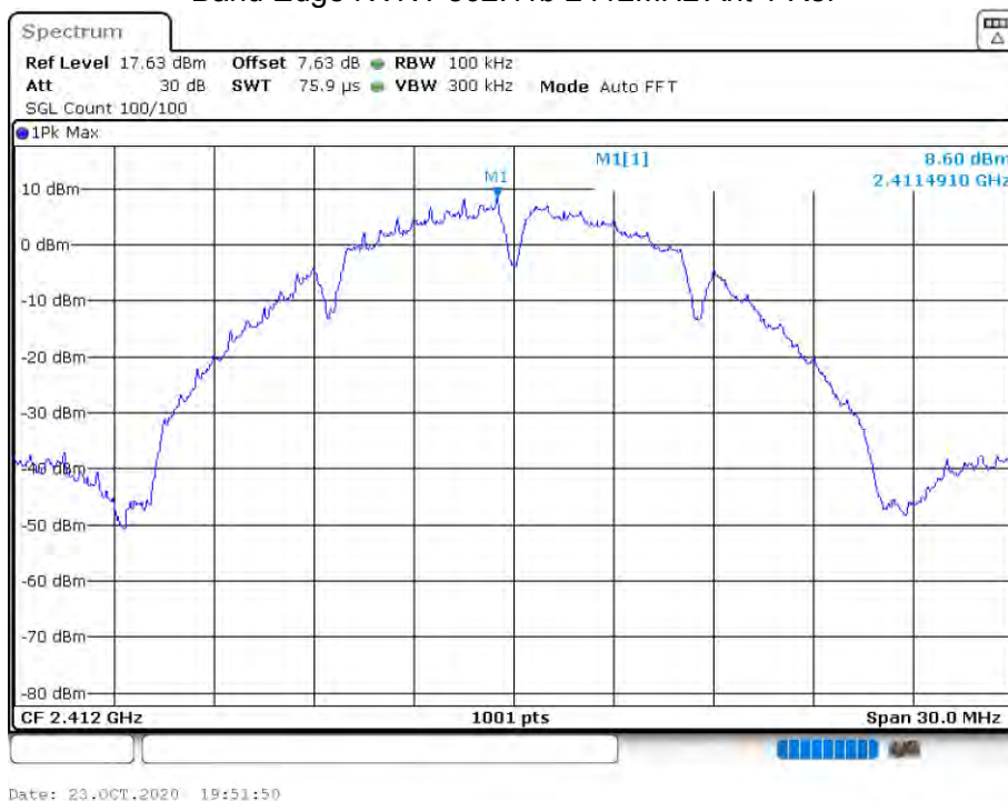
Band Edge NVNT 802.11b 2412MHz Ant 1 Ref
