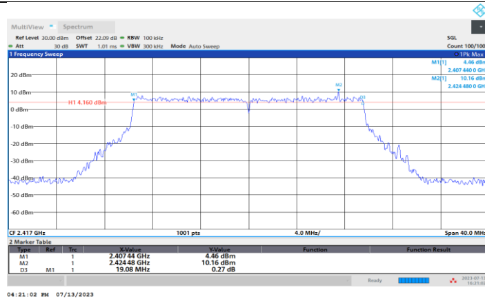
11BE20MIMO_Ant2_2417
