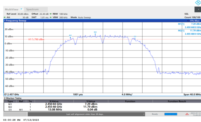
11B-CDD_Ant2_2457
