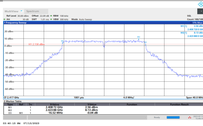
11G-CDD_Ant1_2417
