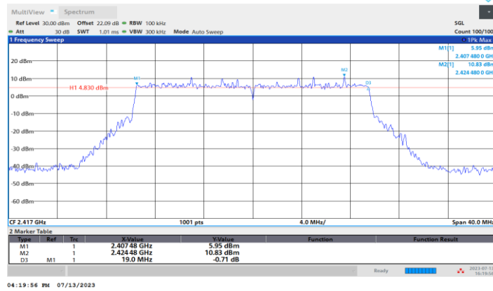
11BE20MIMO_Ant1_2417
