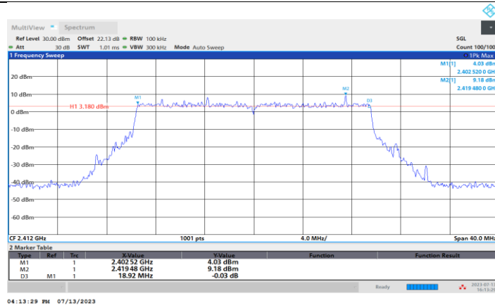
11BE20MIMO_Ant3_2412
