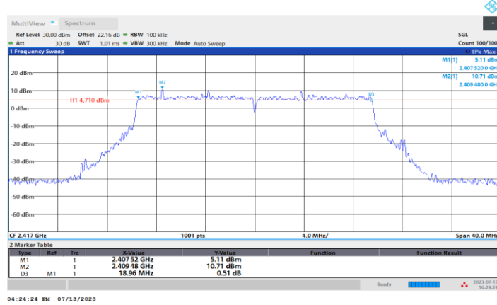
11BE20MIMO_Ant4_2417
