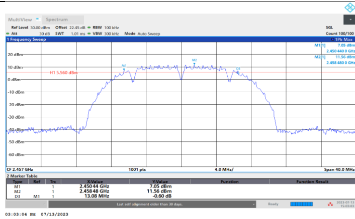
11B-CDD_Ant4_2457
