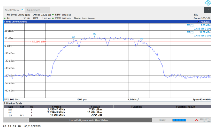
11B-CDD_Ant1_2462
