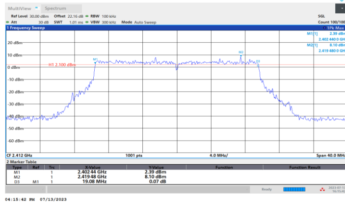
11BE20MIMO_Ant4_2412
