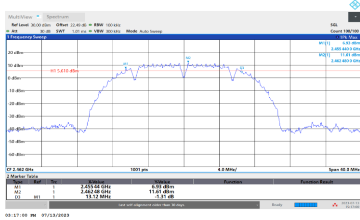
11B-CDD_Ant4_2462
