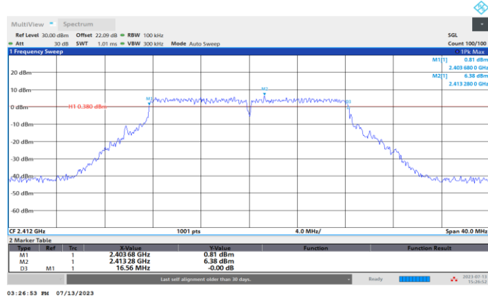
11G-CDD_Ant1_2412
