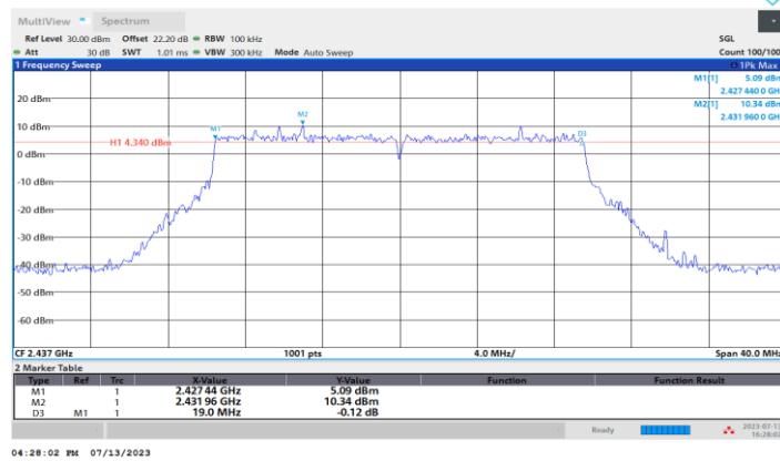
11BE20MIMO_Ant2_2437
