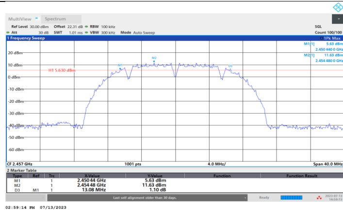
11B-CDD_Ant1_2457
