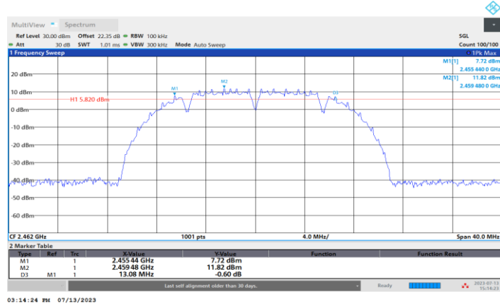
11B-CDD_Ant2_2462
