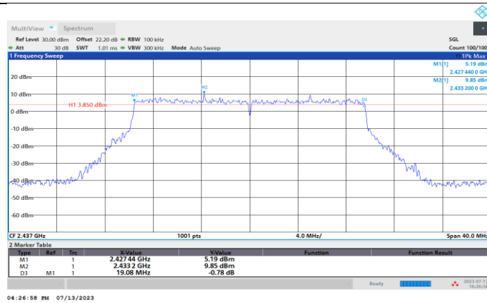
11BE20MIMO_Ant1_2437
