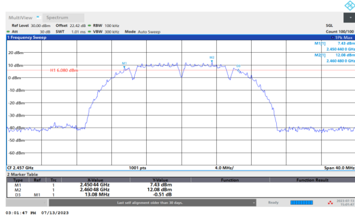
11B-CDD_Ant3_2457
