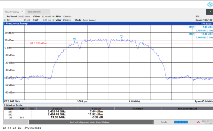
11B-CDD_Ant3_2462
