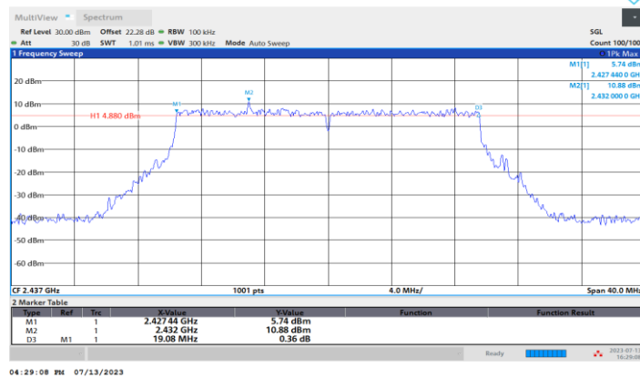
11BE20MIMO_Ant3_2437
