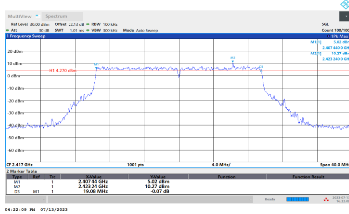
11BE20MIMO_Ant3_2417
