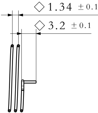
VIEW:B-B
