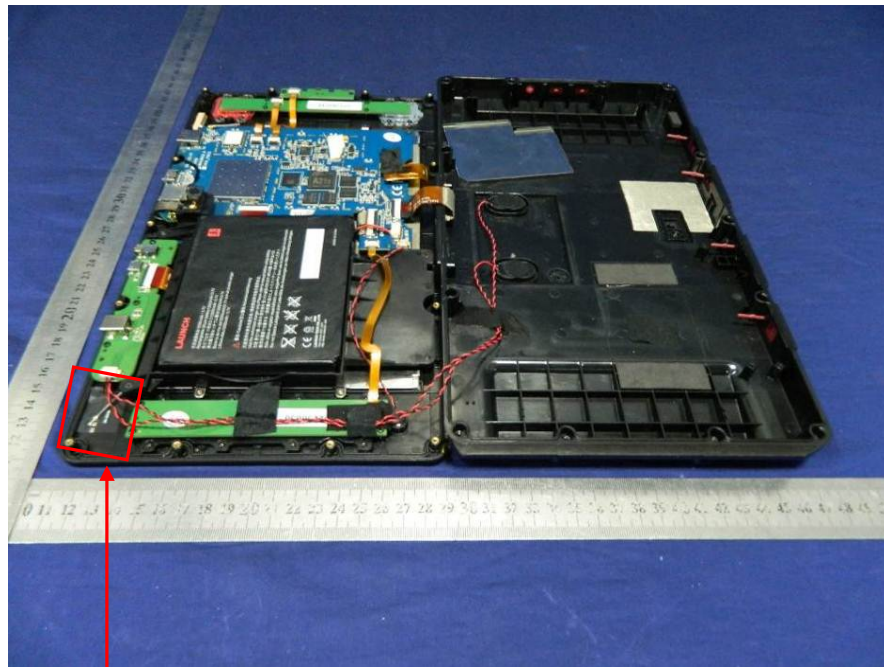
WIFI&BT Antenna
