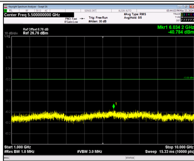
Band12-10MHz-QPSK-23095-1RB#0-Range2:1000~100 00MHz
