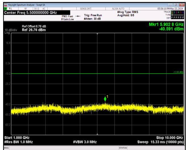
Band13-5MHz-QPSK-23205-1RB#0-Range2:1000~1000 0MHz
