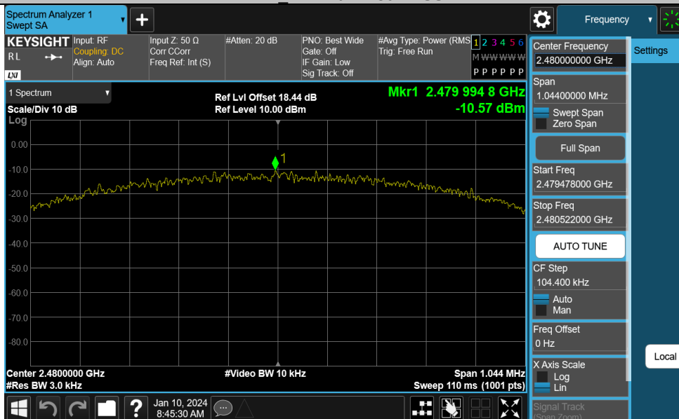
BLE 1M-Ant1-2480-PASS
