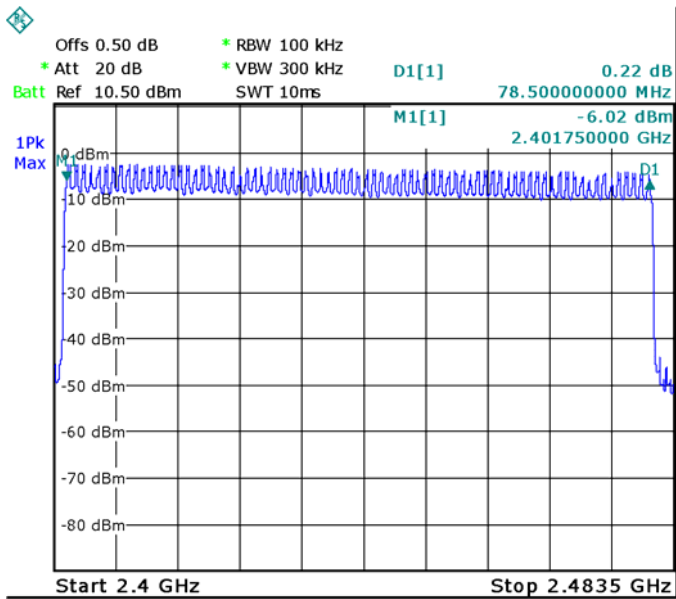
Modulation: \pi/4 DQPSK
