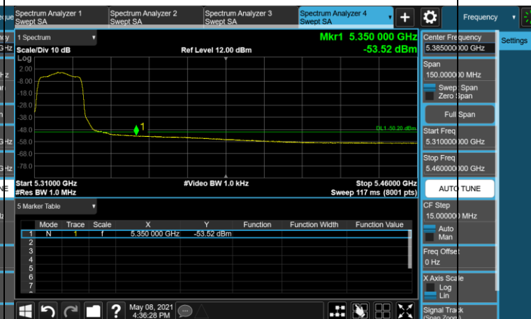
5320MHz with CDD AV
