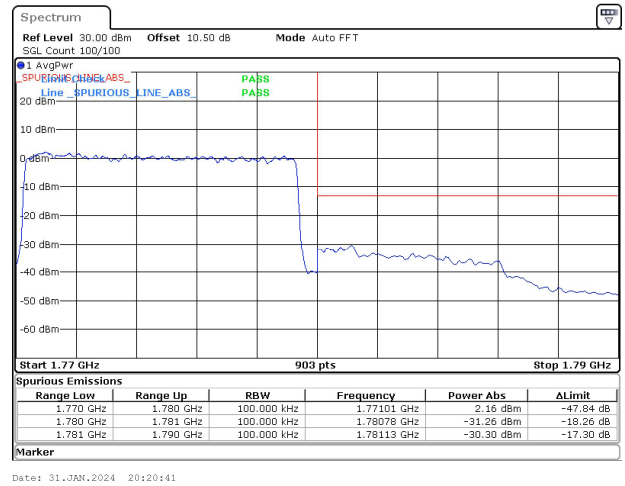
10MHz_15kHz_1775MHz_DFT-s-OFDM QPSK_RB50@0&amp;-30.30 dBm
