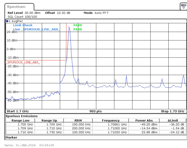
20MHz_15kHz_1720MHz_DFT-s-OFDM QPSK_RB1@0&-14.54 dBm
