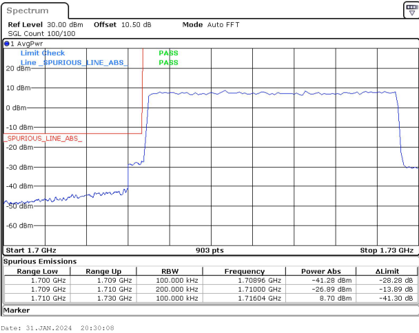
20MHz_15kHz_1720MHz_DFT-s-OFDM QPSK_RB100@0&-26.89 dBm
