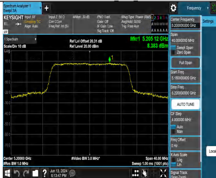
11BE20MIMO_Ant4 5200
