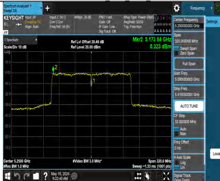
11AX160MIMO_Ant2 5250_UNII-1
