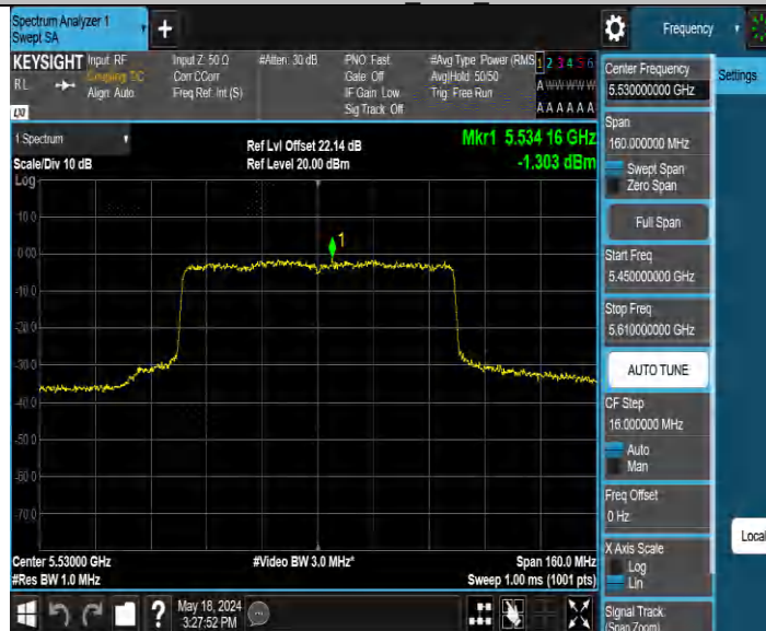
11AX80MIMO_Ant4 5530
