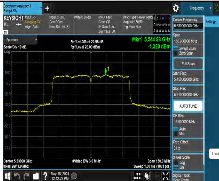
11AC80MIMO_Ant3_5530
