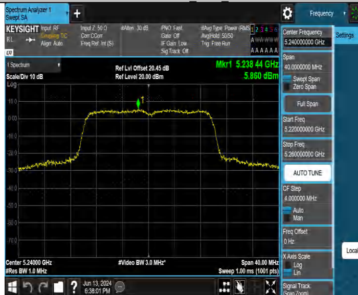
11BE20MIMO_Ant3_5240
