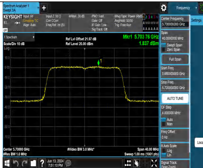
11AX20MIMO_Ant3_5700
