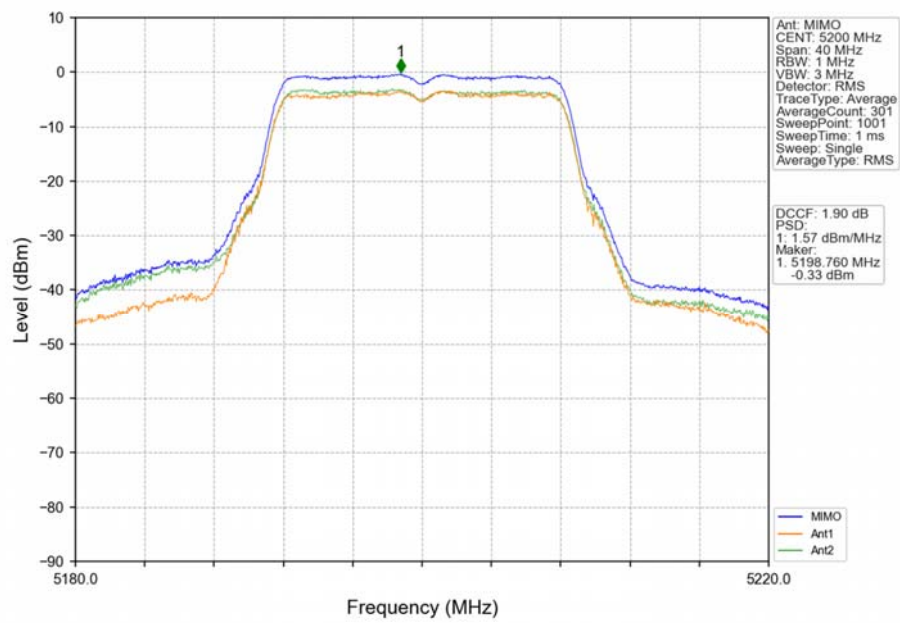
802.11a_MCH_5200MHz_MIMO_NTNV
