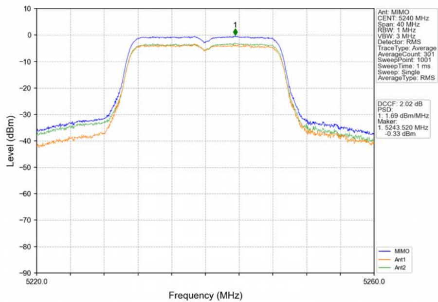
802.11n(HT20)_HCH_5240MHz_MIMO_NTNV
