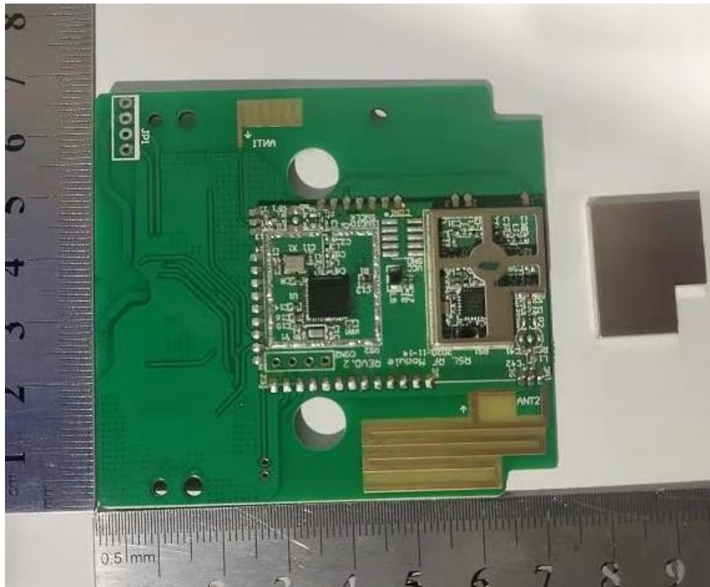
PCBA of 5E22E9
