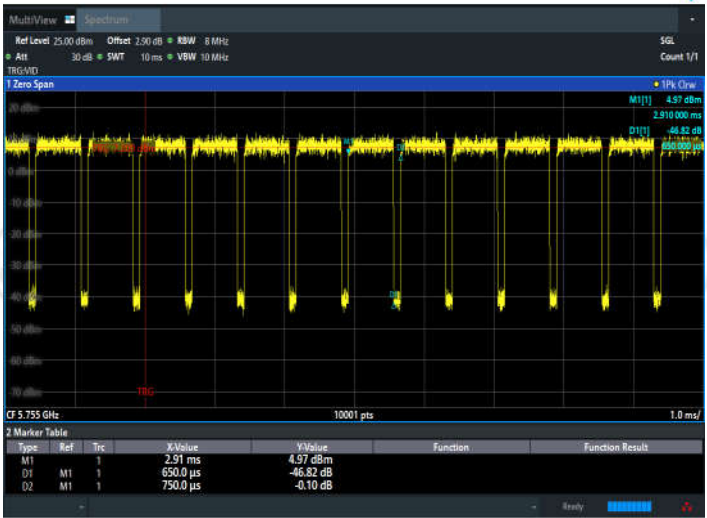
11N40SISO_Ant2_5755
