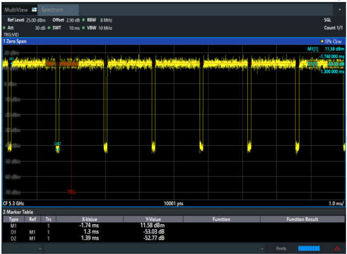
11N20SISO_Ant2_5300
