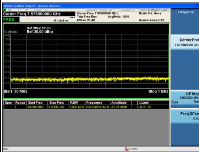
CSE_MIMO(ANT5)_n77(K)_30KHz_256QAM_20M CH633334_1RB@1
