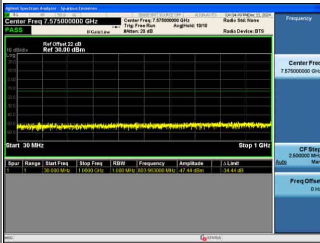
CSE_MIMO(ANT5)_n77(K)_30KHz_256QAM_15M CH633334_1RB@1
