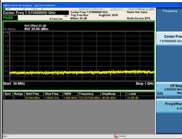
CSE_MIMO(ANT5)_n77(K)_30KHz_256QAM_40M CH633334_1RB@1
