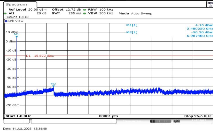
BLE_1M_Ant2_2480_1000~26500
