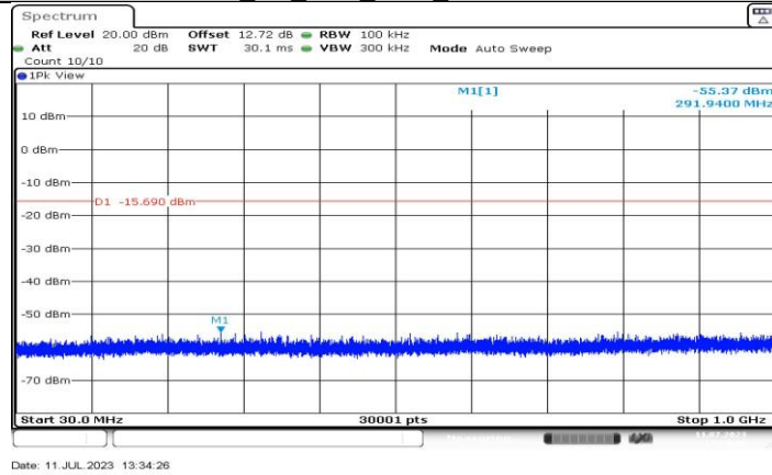
BLE_1M_Ant2_2480_30~1000
