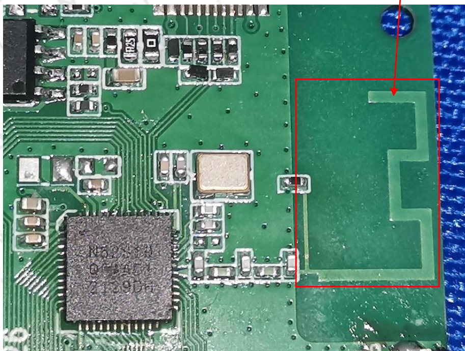
BLE Antenna
