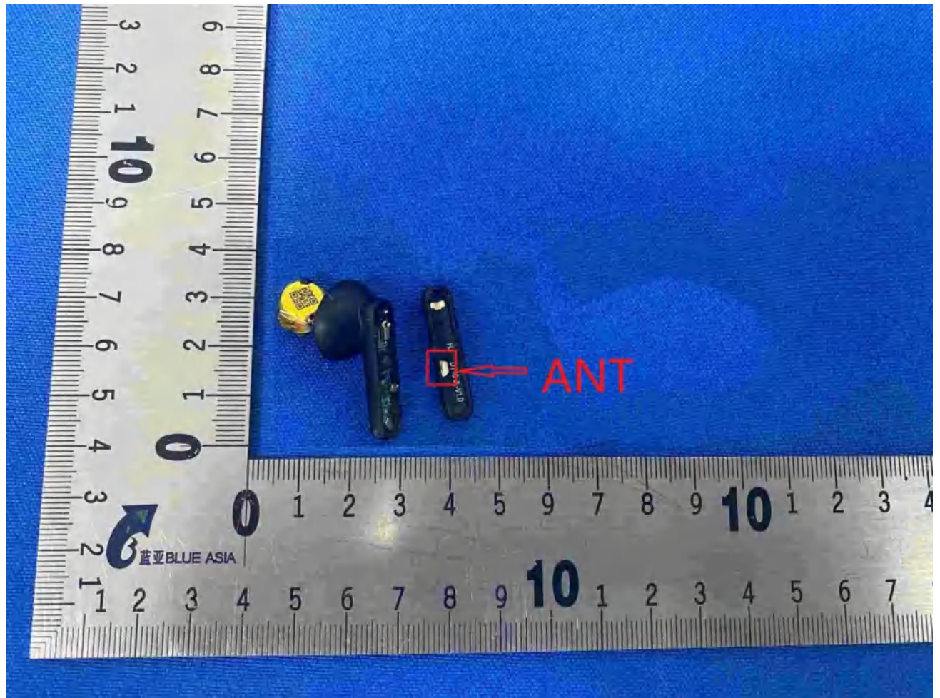
EUT Antenna
