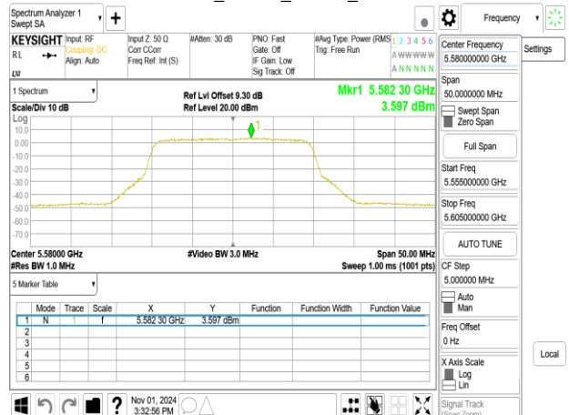
802.11ax_20MHz_Chain1_5580MHz
