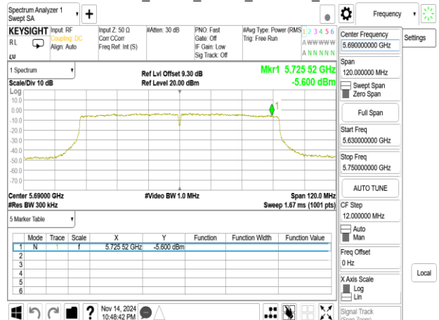
802.11ac_80MHz_Chain0_5690MHz_UNII 3
