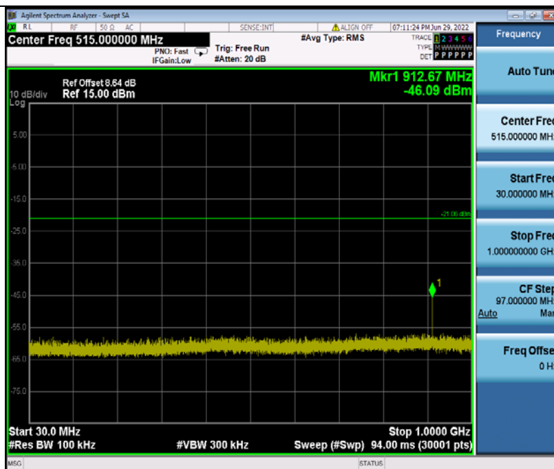
DH5 Ant1_2480_30~1000
