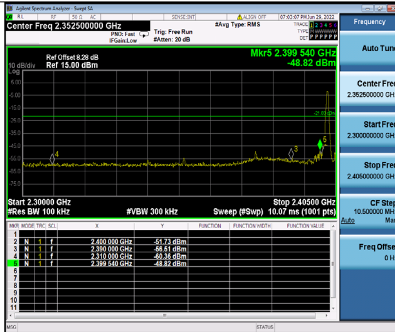
DH5_Ant1_Low_2402
