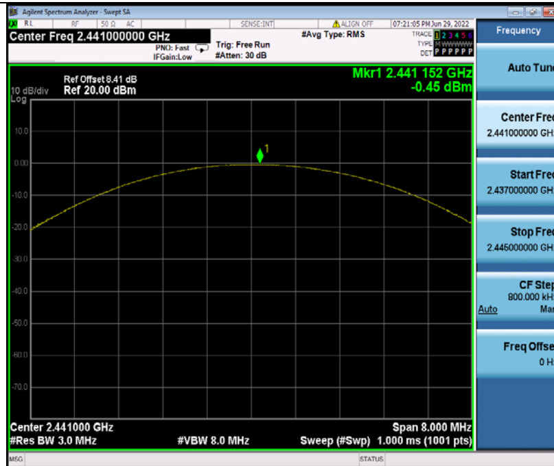
2DH5 Ant1 2441
