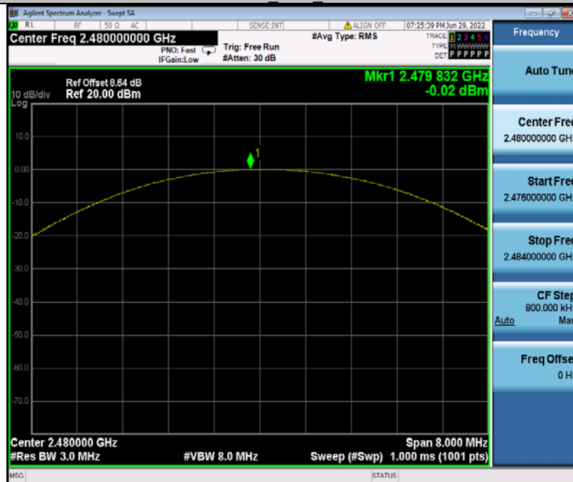
2DH5 Ant1 2480
