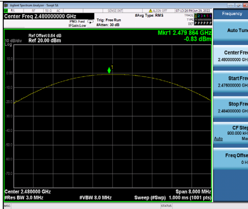
DH5_Ant1_2480
