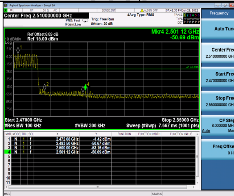
DH5 Ant1 High Hop 2480
