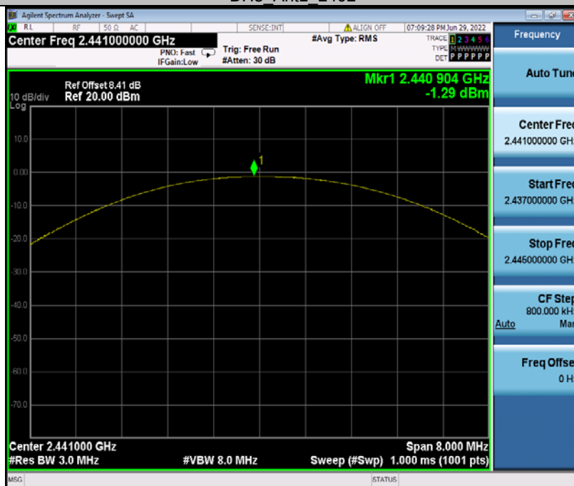
DH5_Ant1_2441
