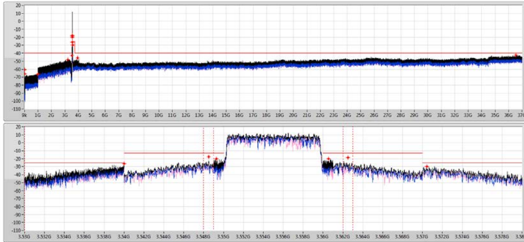
Band 48_10MHz_2TX 3555MHz_QPSK
