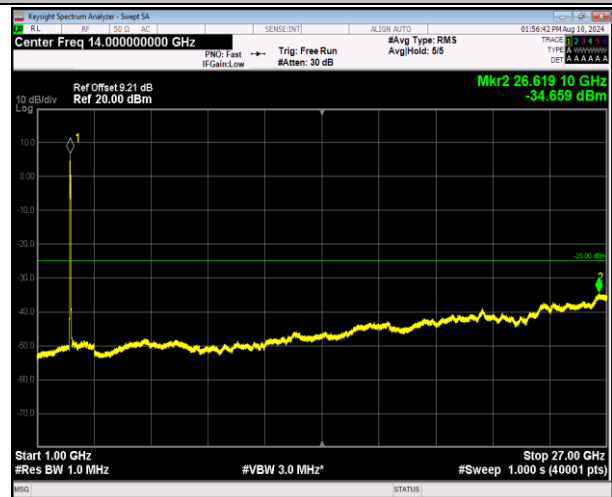
7-7-20MHz-20MHz-QPSK-QPSK-20850-21048-100RB#0-1 00RB#0-1000~27000MHz-PASS
