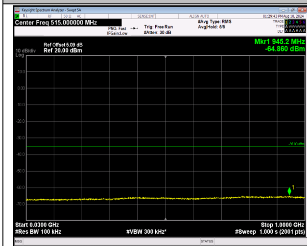
7-7-20MHz-10MHz-QPSK-QPSK-21251-21395-1RB#99-0RB#0-30~1000MHz-PASS
