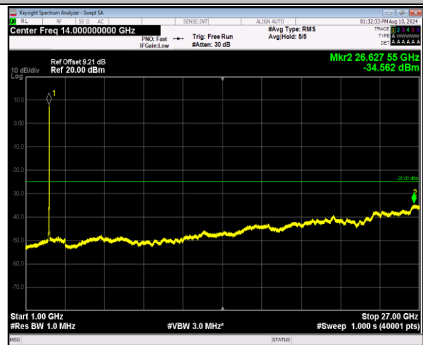
7-7-20MHz-10MHz-QPSK-QPSK-21251-21395-100RB#0-50RB#0-1000~27000MHz-PASS
