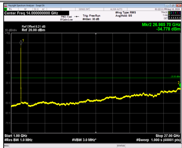
7-7-20MHz-10MHz-QPSK-QPSK-20850-20994-100RB#0-50RB#0-1000~27000MHz-PASS
