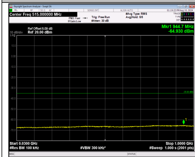
7-7-20MHz-10MHz-QPSK-QPSK-20850-20994-1RB#99-0RB#0-30~1000MHz-PASS
