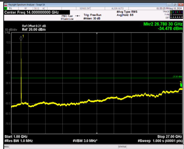
7-7-20MHz-20MHz-QPSK-QPSK-20850-21048-1RB#0-1RB #99-1000~27000MHz-PASS
