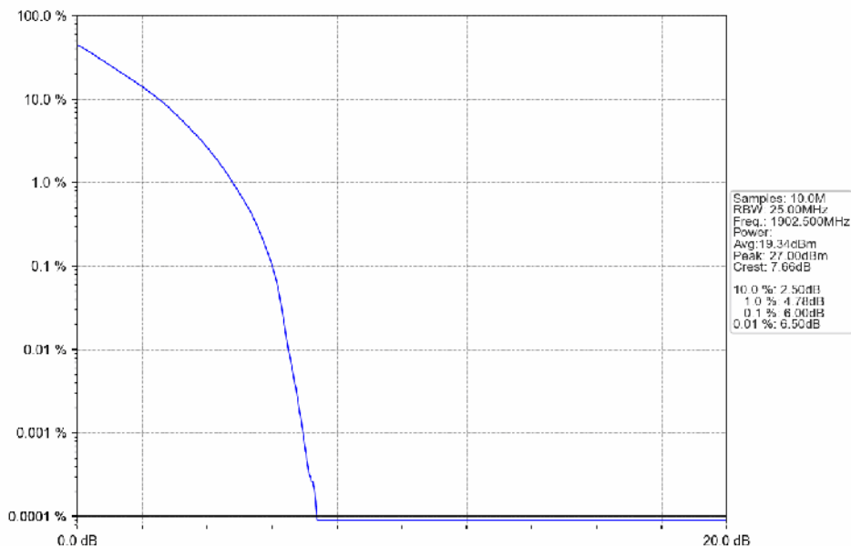
Band2 15MHz QPSK HCH 1902.5MHz RB 75 0 NTNV
