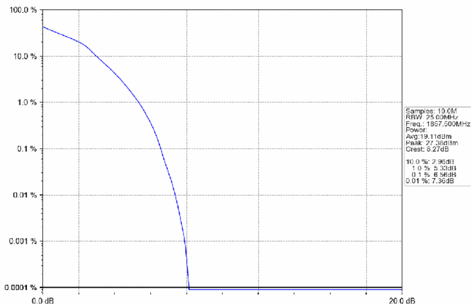
Band2 15MHz 16QAM LCH 1857.5MHz RB 75 0 NTNV
