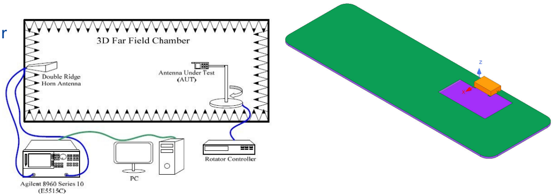
Fig.2 暗室示意图
