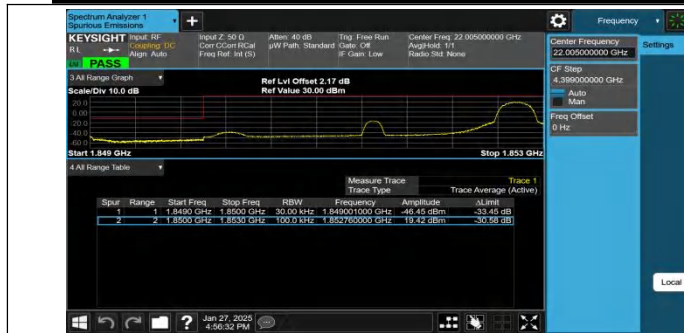
Band2-3MHz-QPSK-18615-1RB#14-PASS
