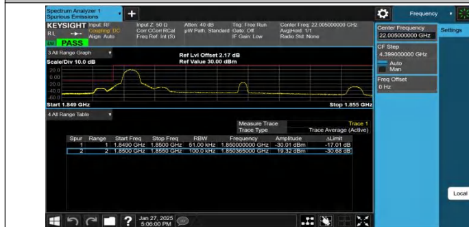
Band2-5MHz-QPSK-18625-1RB#0-PASS
