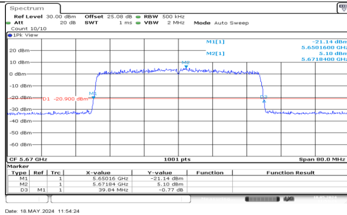
11AX40MIMO_Ant1_5670
