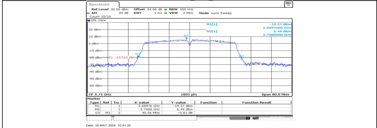
11N40MIMO_Ant2_5710
