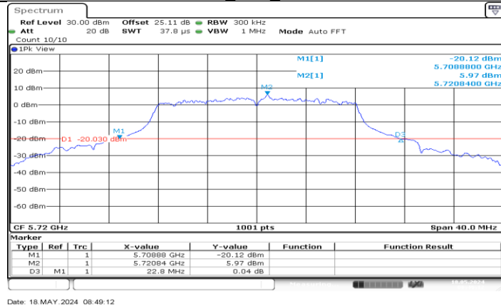
11A Ant2 5720
