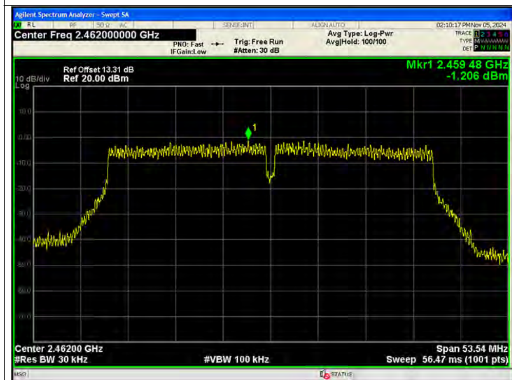
PSD NVNT n40 2462MHz Ant1
