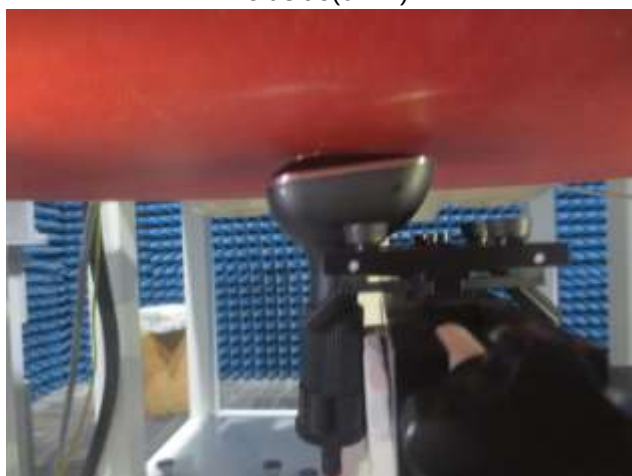
Top side(0mm)
