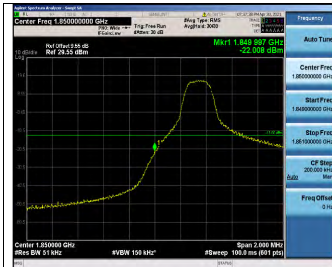
Band2-5MHz-16QAM-18625-1RB#0
