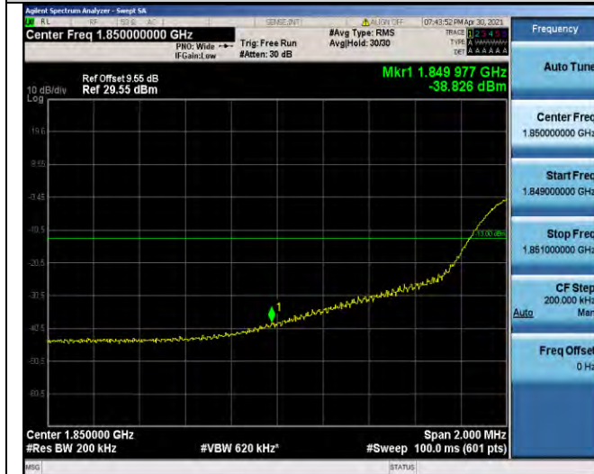
Band2-20MHz-16QAM-18700-100RB#0
