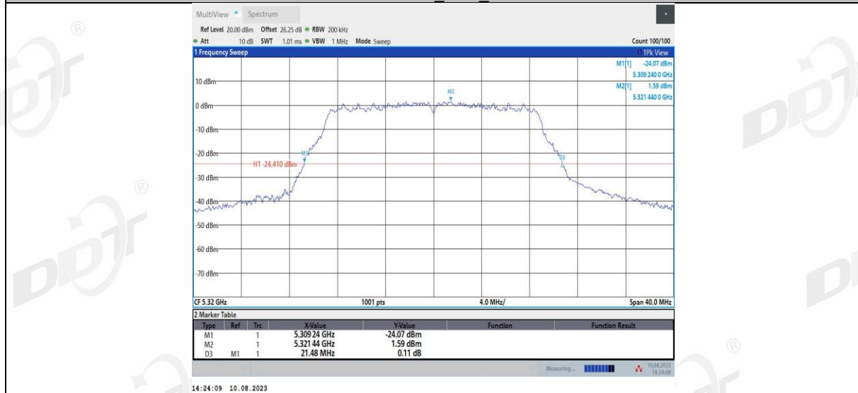
11N20MIMO_Ant2_5320
