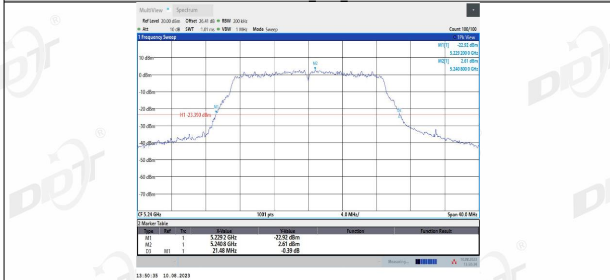
11N20MIMO_Ant2_5240
