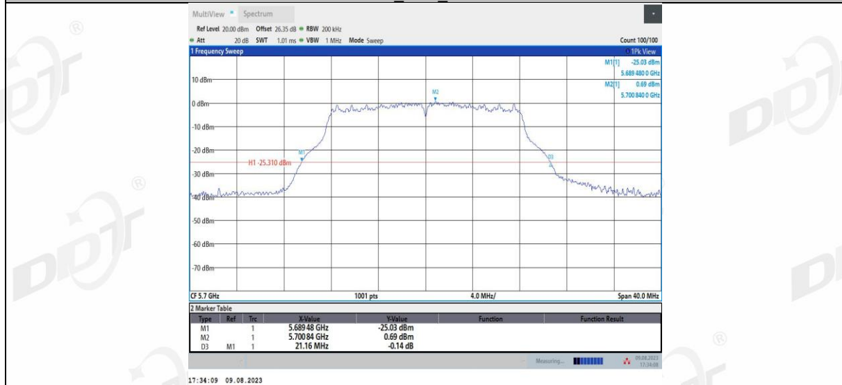
11A_Ant2_5700
