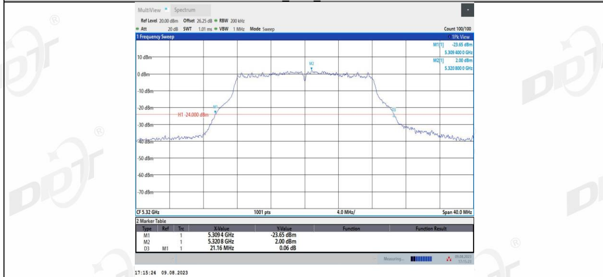
11A_Ant2_5320
