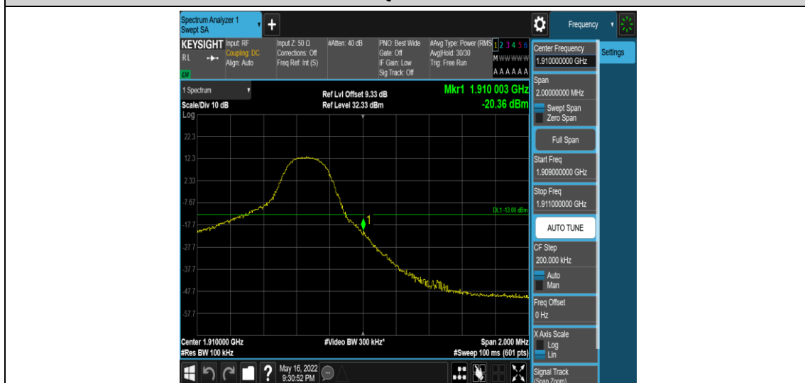
Band2-5MHz-QPSK-19175-1RB#24
