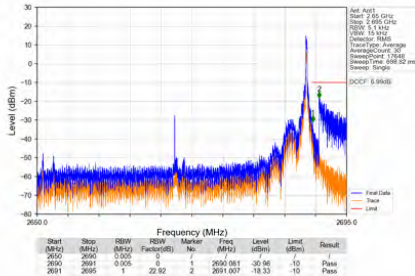
n41_15kHz_SISO_NTNV_40MHz_CP-OFDM_QPSK_2670MHz_Inner_1RB_Right
