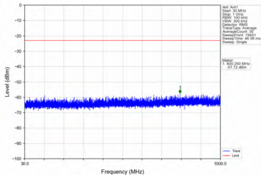
n41_15kHz_SISO_NTNV_40MHz_CP-OFDM QPSK_2516.01MHz_Edge_1RB_Left
