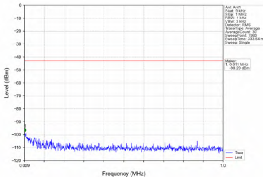
n41_15kHz_SISO_NTNV_40MHz_DFT-s-OFDM_PI/2_BPSK_2670MHz_Inner_1RB_Right
