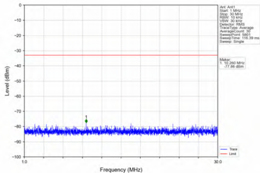
n41_15kHz_SISO_NTNV_40MHz_DFT-s-OFDM_PI/2_BPSK_2670MHz_Inner_1RB_Right
