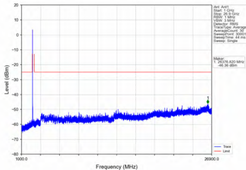
n41_15kHz_SISO_NTNV_40MHz_CP-OFDM QPSK_2593.005MHz_Edge_1RB_Left
