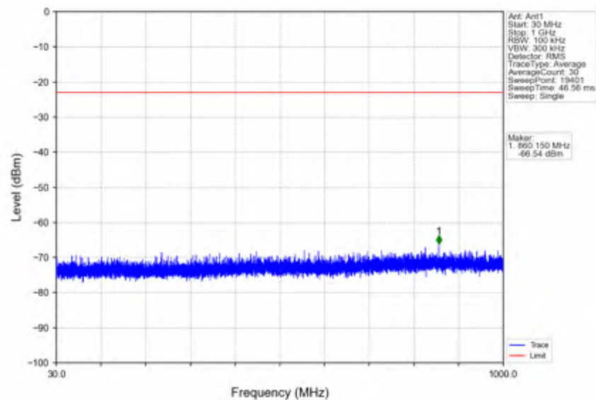
n41_15kHz_SISO_NTNV_40MHz_DFT-s-OFDM_PI/2_BPSK_2670MHz_Inner_1RB_Right
