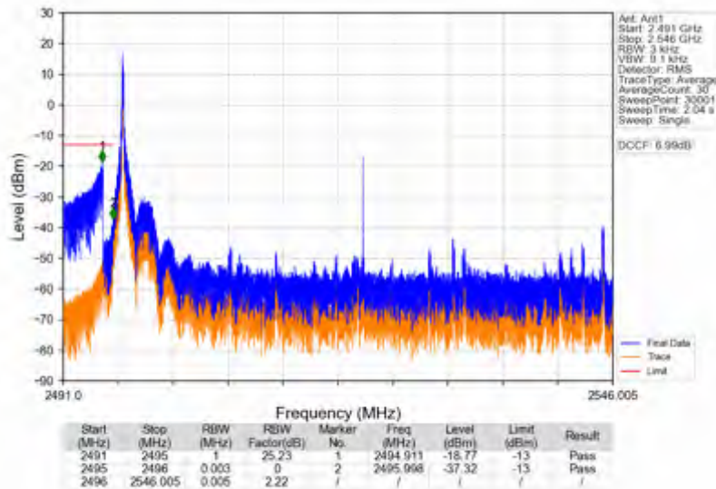
n41_15kHz_SISO_NTNV_50MHz_DFT-s-OFDM QPSK_2521.005MHz_Inner_1RB_Left
