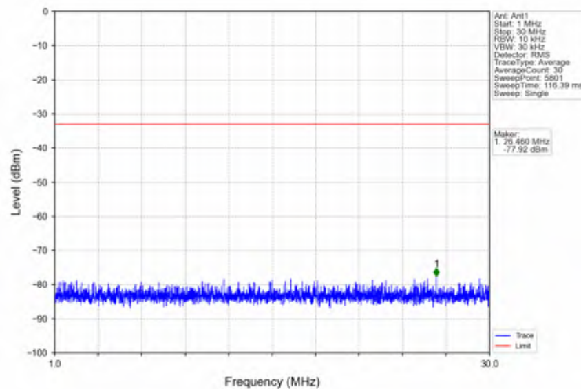
n41_30kHz_SISO_NTNV_10MHz_CP-OFDM_QPSK_2685MHz_Inner_1RB_Right
