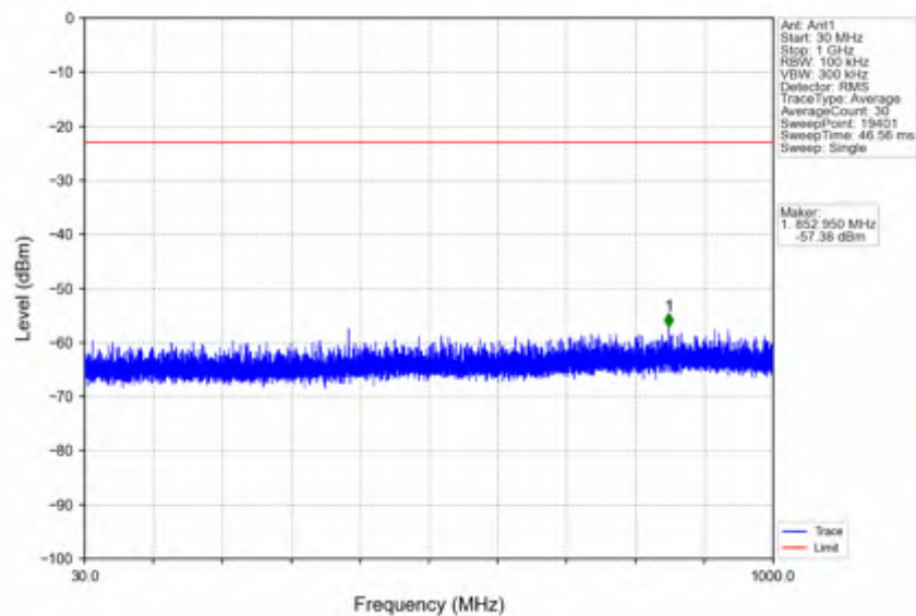
n41_15kHz_SISO_NTNV_50MHz_CP-OFDM QPSK_2593.005MHz_Edge_1RB_Left
