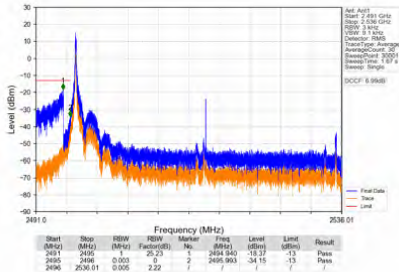
n41_15kHz_SISO_NTNV_40MHz_CP-OFDM_QPSK_2516.01MHz_Inner_1RB_Left
