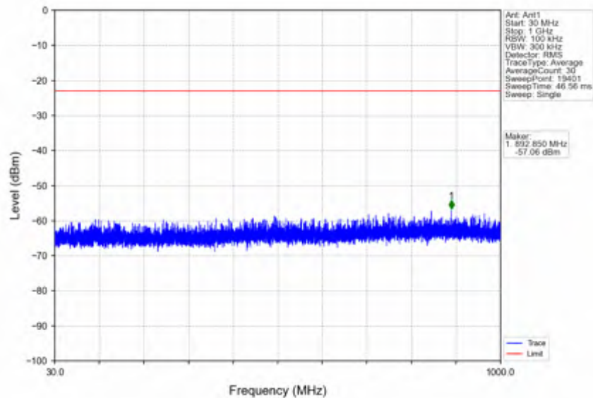
n41_15kHz_SISO_NTNV_40MHz_CP-OFDM QPSK_2593.005MHz_Edge_1RB_Left
