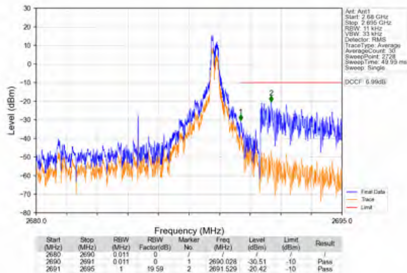
n41_30kHz_SISO_NTNV_10MHz_CP-OFDM QPSK_2685MHz_Inner_1RB_Right
