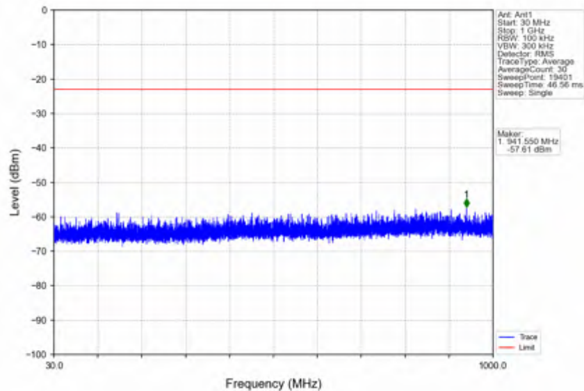
n41_15kHz_SISO_NTNV_50MHz_DFT-s-OFDM QPSK_2521.005MHz_Edge_1RB_Left
