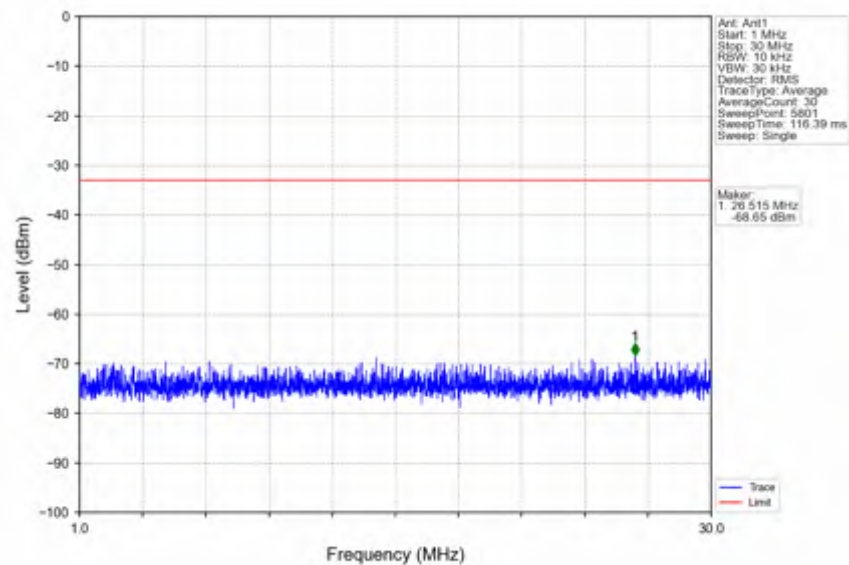
n41_15kHz_SISO_NTNV_40MHz_CP-OFDM QPSK_2516.01MHz_Edge_1RB_Left
