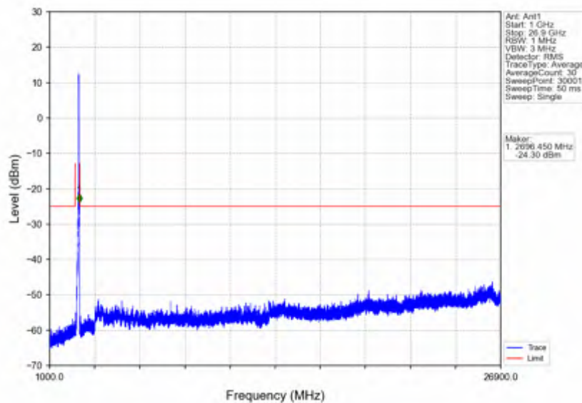
n41_15kHz_SISO_NTNV_40MHz_DFT-s-OFDM QPSK_2670MHz_Inner_1RB_Right
