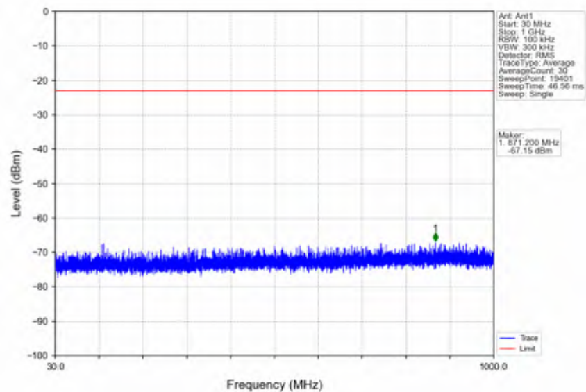
n41_15kHz_SISO_NTNV_40MHz_CP-OFDM QPSK_2670MHz_Inner_1RB_Right
