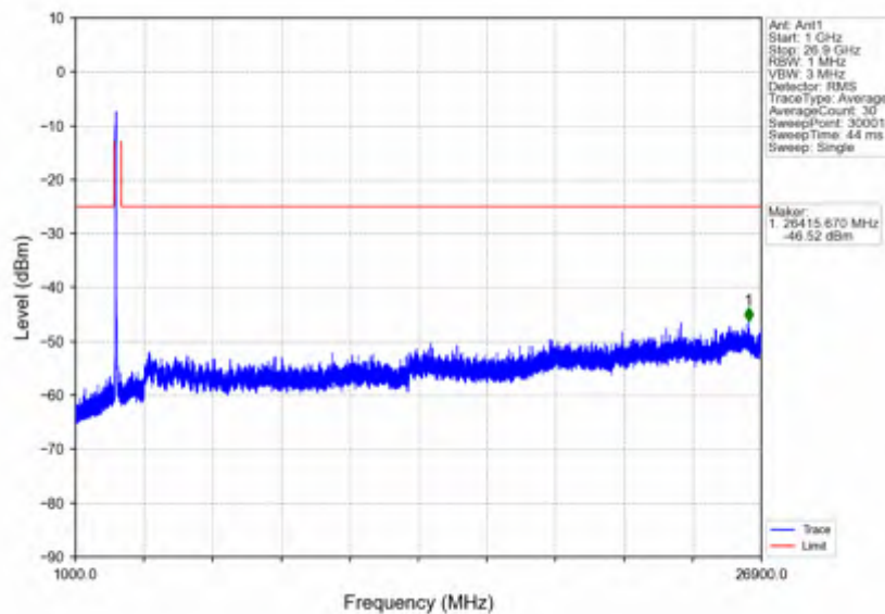
n41_15kHz_SISO_NTNV_40MHz_DFT-s-OFDM QPSK_2516.01MHz_Inner_1RB_Left
