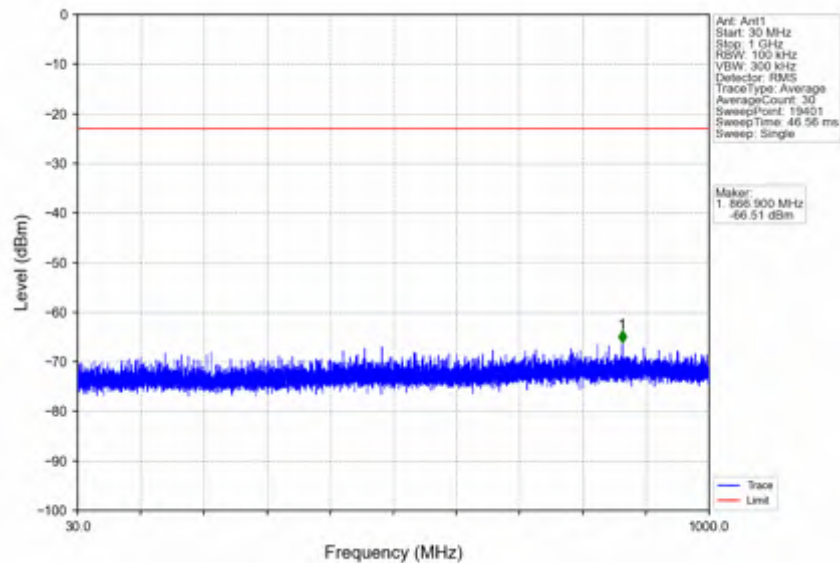
n41_15kHz_SISO_NTNV_50MHz_DFT-s-OFDM QPSK_2521.005MHz_Inner_1RB_Left
