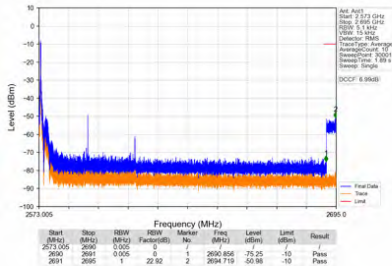
n41_15kHz_SISO_NTNV_40MHz_CP-OFDM QPSK_2593.005MHz_Edge_1RB_Left
