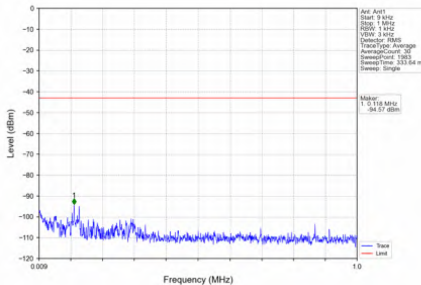
n41_30kHz_SISO_NTNV_15MHz_DFT-s-OFDM_PI/2_BPSK_2503.5MHz_Inner_1RB_Left
