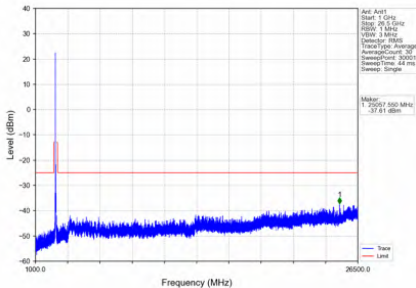
n41_15kHz_SISO_NTNV_50MHz_CP-OFDM QPSK_2593.005MHz_Edge_1RB_Left
