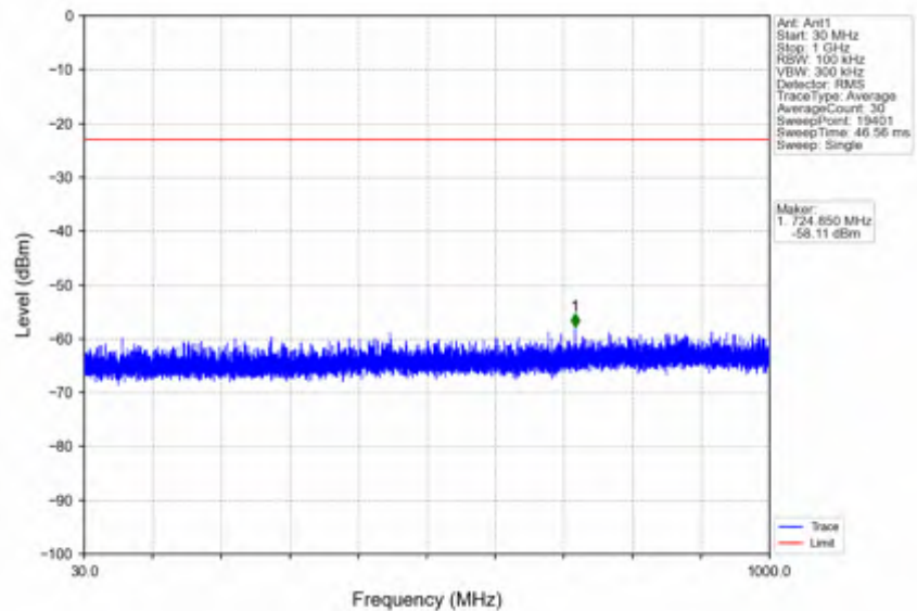
n41_15kHz_SISO_NTNV_50MHz_CP-OFDM QPSK_2521.005MHz_Edge_1RB_Left
