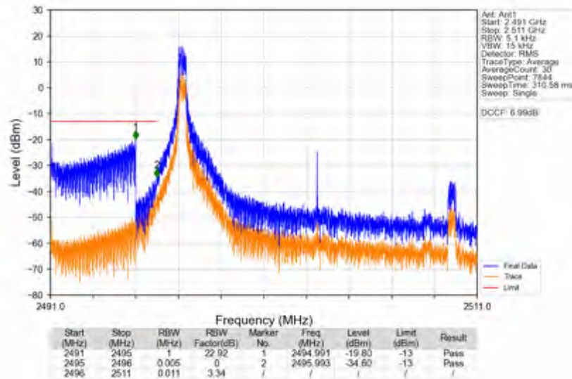
n41_30kHz_SISO_NTNV_15MHz_DFT-s-OFDM_PI/2_BPSK_2503.5MHz_Inner_1RB_Left
