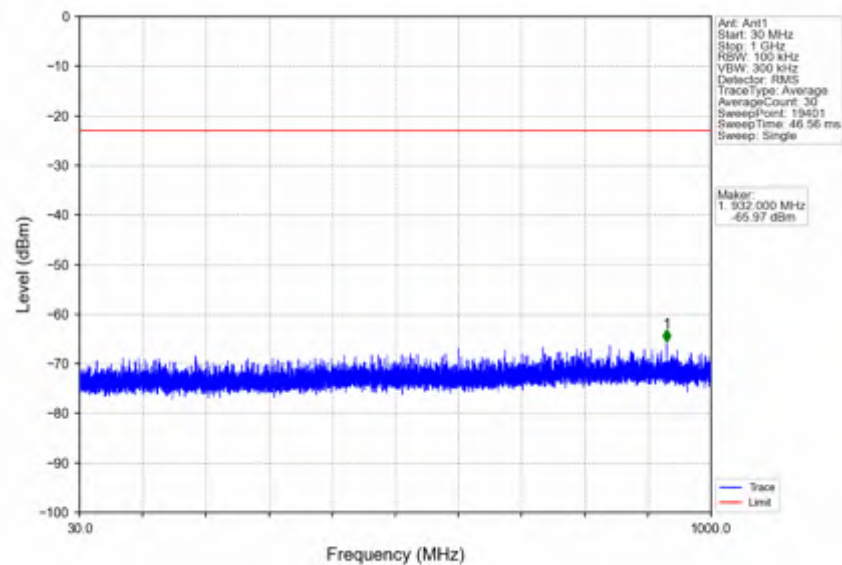
n41_15kHz_SISO_NTNV_50MHz_CP-OFDM QPSK_2521.005MHz_Inner_1RB_Left
