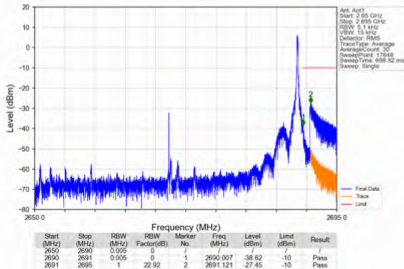
n41_15kHz_SISO_NTNV_40MHz_DFT-s-OFDM QPSK_2670MHz_Inner_1RB_Right
