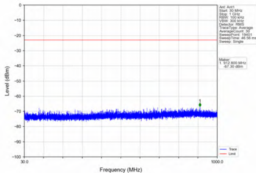
n41_15kHz_SISO_NTNV_40MHz_DFT-s-OFDM_QPSK_2670MHz_Inner_1RB_Right
