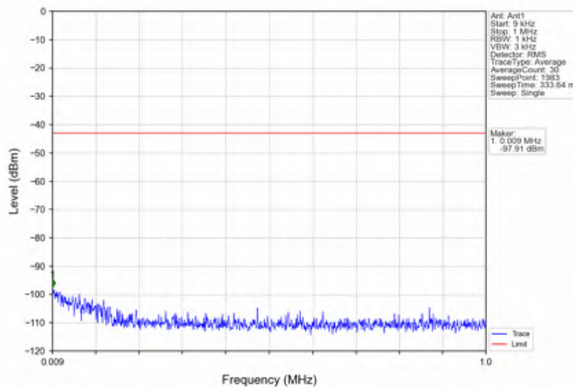
n41_15kHz_SISO_NTNV_40MHz_CP-OFDM_QPSK_2516.01MHz_Inner_1RB_Left
