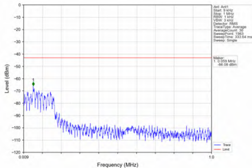
n41_15kHz_SISO_NTNV_50MHz_DFT-s-OFDM QPSK_2521.005MHz_Edge_1RB_Left
