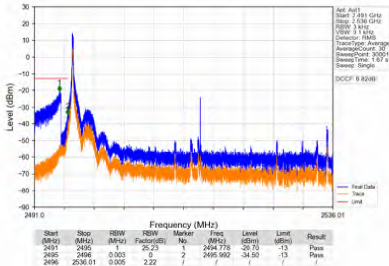
n41_15kHz_SISO_NTNV_40MHz_DFT-s-OFDM QPSK_2516.01MHz_Inner_1RB_Left
