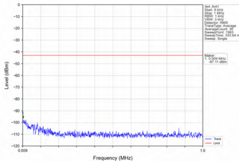
n41_15kHz_SISO_NTNV_40MHz_CP-OFDM_QPSK_2670MHz_Inner_1RB_Right
