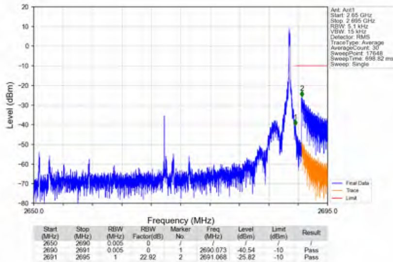
n41_15kHz_SISO_NTNV_40MHz_DFT-s-OFDM_PI/2_BPSK_2670MHz_Inner_1RB_Right
