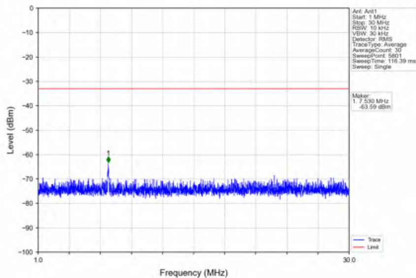
n41_15kHz_SISO_NTNV_50MHz_CP-OFDM QPSK_2593.005MHz_Edge_1RB_Left
