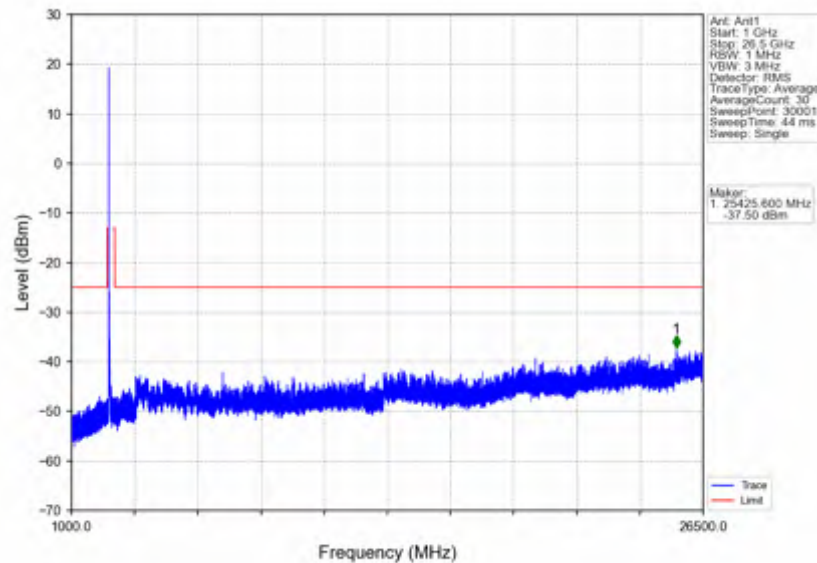
n41_15kHz_SISO_NTNV_50MHz_DFT-s-OFDM QPSK_2521.005MHz_Edge_1RB_Left
