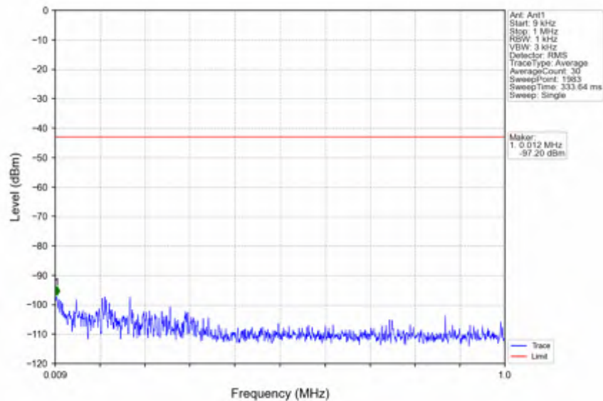
n41_30kHz_SISO_NTNV_10MHz_DFT-s-OFDM QPSK_2685MHz_Inner_1RB_Right
