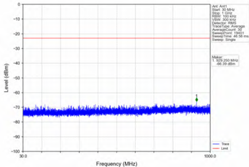
n41_30kHz_SISO_NTNV_10MHz_DFT-s-OFDM QPSK_2685MHz_Inner_1RB_Right
