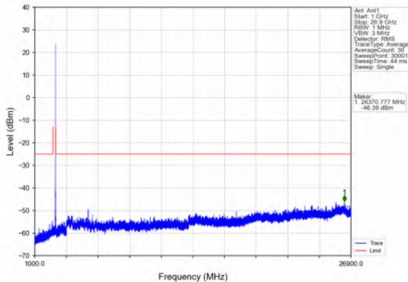
n41_30kHz_SISO_NTNV_10MHz_DFT-s-OFDM QPSK_2685MHz_Inner_1RB_Right
