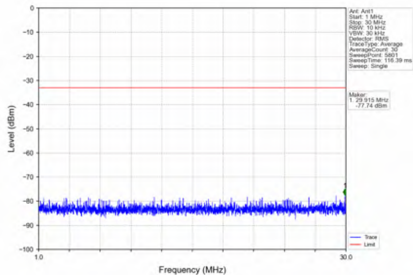
n41_15kHz_SISO_NTNV_40MHz_DFT-s-OFDM_QPSK_2516.01MHz_Inner_1RB_Left
