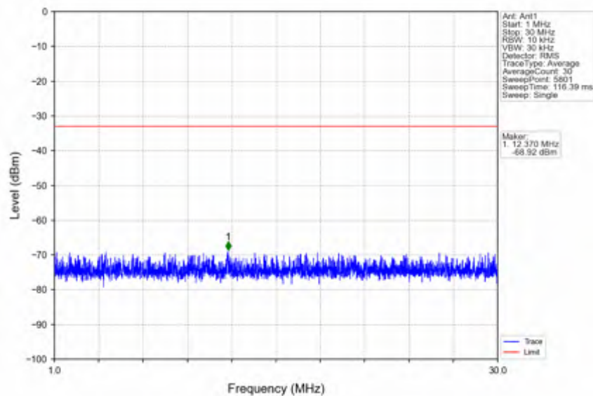
n41_15kHz_SISO_NTNV_40MHz_DFT-s-OFDM QPSK_2593.005MHz_Edge_1RB_Left
