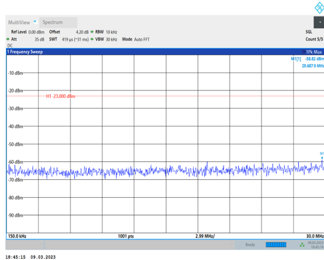
Band66-20MHz-QPSK-132072-1RB#0-Range2:0.15~30MHz
