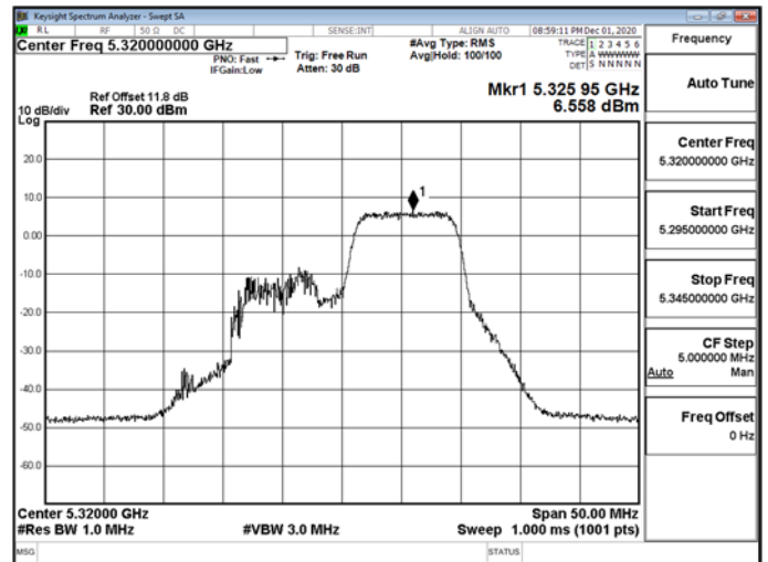
802.11ax_20MHz_RU_26_8_5320MHz-5320
