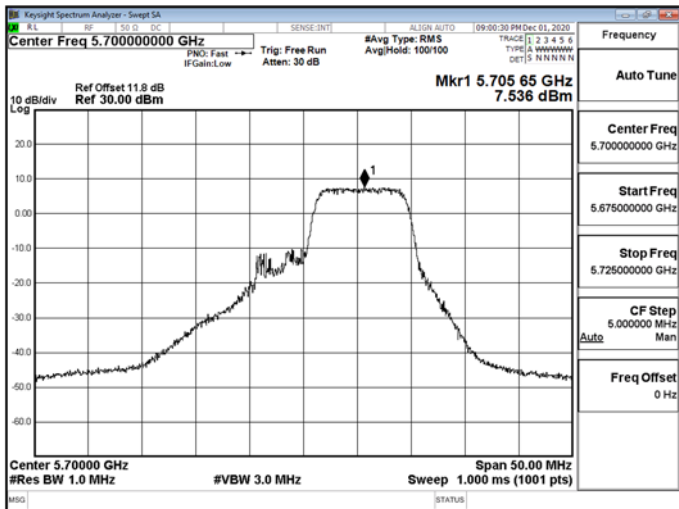
802.11ax_20MHz_RU_26_8_5700MHz-5700
