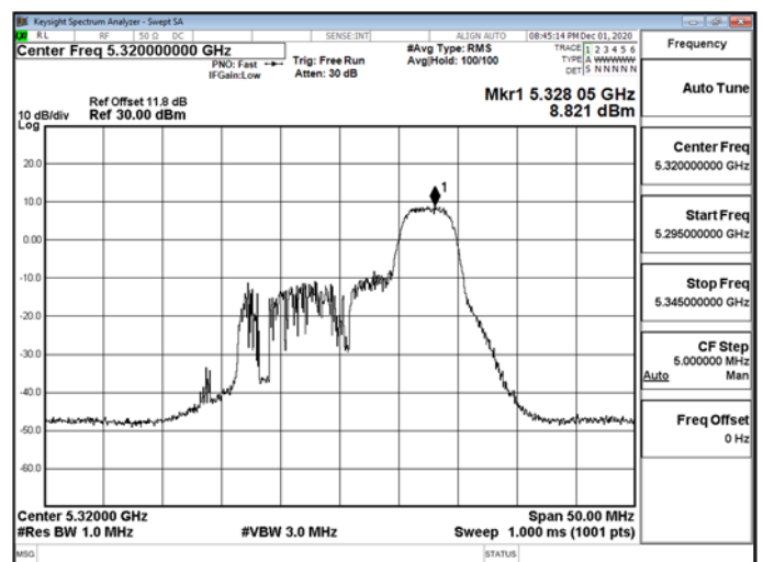
802.11ax_20MHz_RU_52_40_5320MHz-5320
