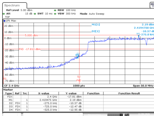
BE-NR, SISO-B, 802.11ax40-HE0, Ch1
