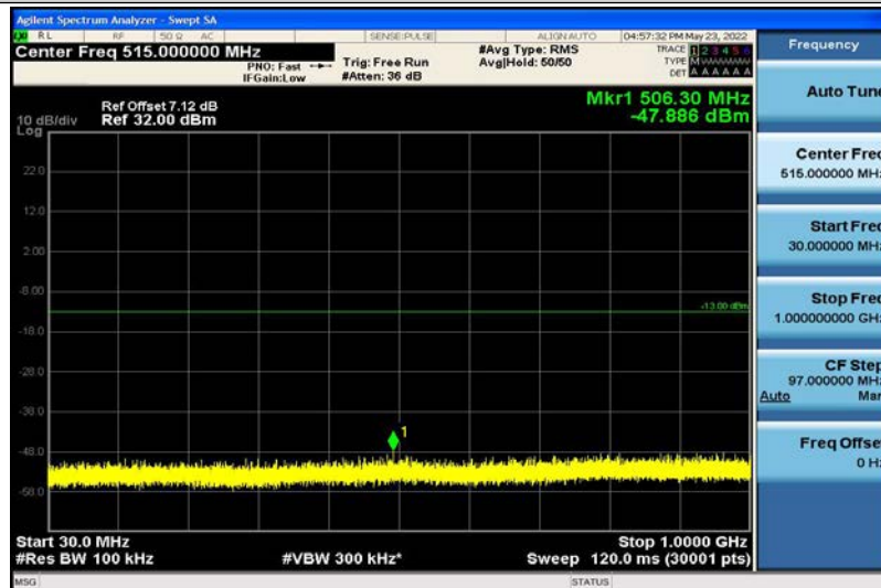
Band2-3MHz-QPSK-19185-1RB#0-30~1000MHz
