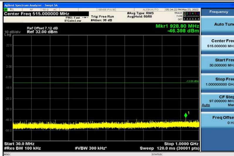
Band2-10MHz-QPSK-19150-1RB#0-30~1000MHz
